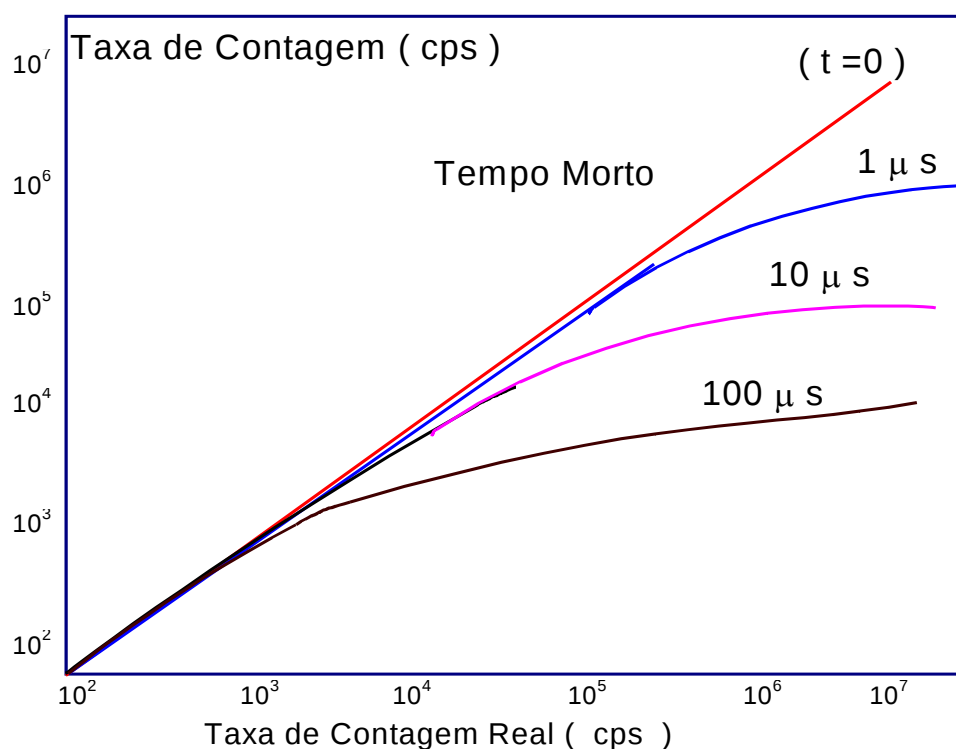
Figura 4.1 Taxa de contagem observada como função da taxa de contagem real, para detectores com 1 \mu s, 10 \mu s e 100 \mu s de tempo morto. (Adaptado de “Introductory Physics of Nuclear Medicine”, Ramesh Chandra - New York University Medical School, NY, 1976. )
