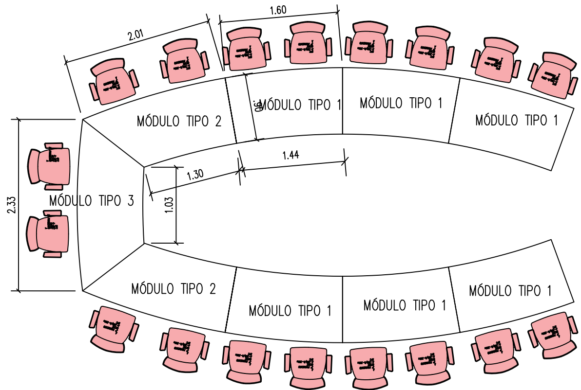
PLANTA MESA REUNIÕES
