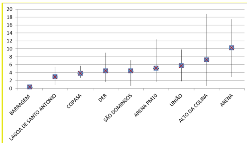
Gráfico 2. Concentrações mínimas, médias e máximas de arsênio ( \text{ng/m}^3 ) no material particulado atmosférico*, relativas ao período de maio de 2011 a junho de 2012, nas 8 estações de amostragem localizadas no município de Paracatu.
