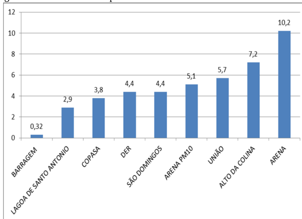
Gráfico 1. Concentrações médias de arsênio ( \text{ng/m}^3 ) no material particulado atmosférico*, relativas ao período de maio de 2011 a junho de 2012, nas 8 estações de amostragem localizadas no município de Paracatu.
