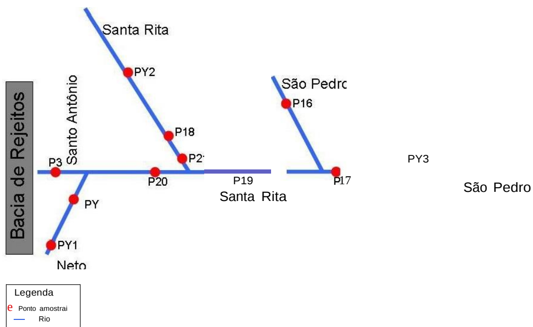
Figura 6. Posicionamento esquemático das estações de amostragem ao longo das sub-bacias do eixo hidrográfico de saída da Bacia de Rejeito.
