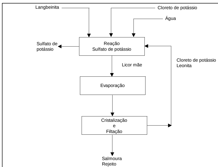
Figura 4 - Diagrama esquemático da produção de sulfato de potássio a partir da langbeinita.
