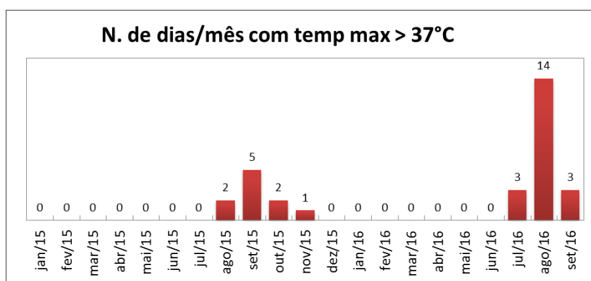
Figura 9. Número de dias por mês com temperatura máxima registrada acima de 37 °C entre os anos de 2015 e 2016 na estação meteorológica de Rio Branco-AC. Fonte dos dados: Instituto Nacional de Meteorologia (INMET).
