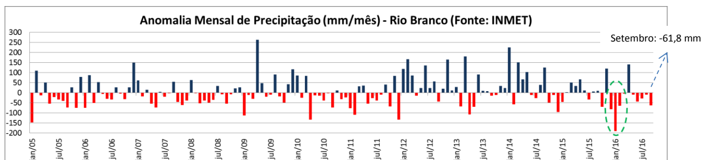
Figura 7. Anomalia mensal de precipitação entre os anos de 2005 e 2016 na estação meteorológica de Rio Branco-AC. Fonte dos dados: Instituto Nacional de Meteorologia (INMET).
