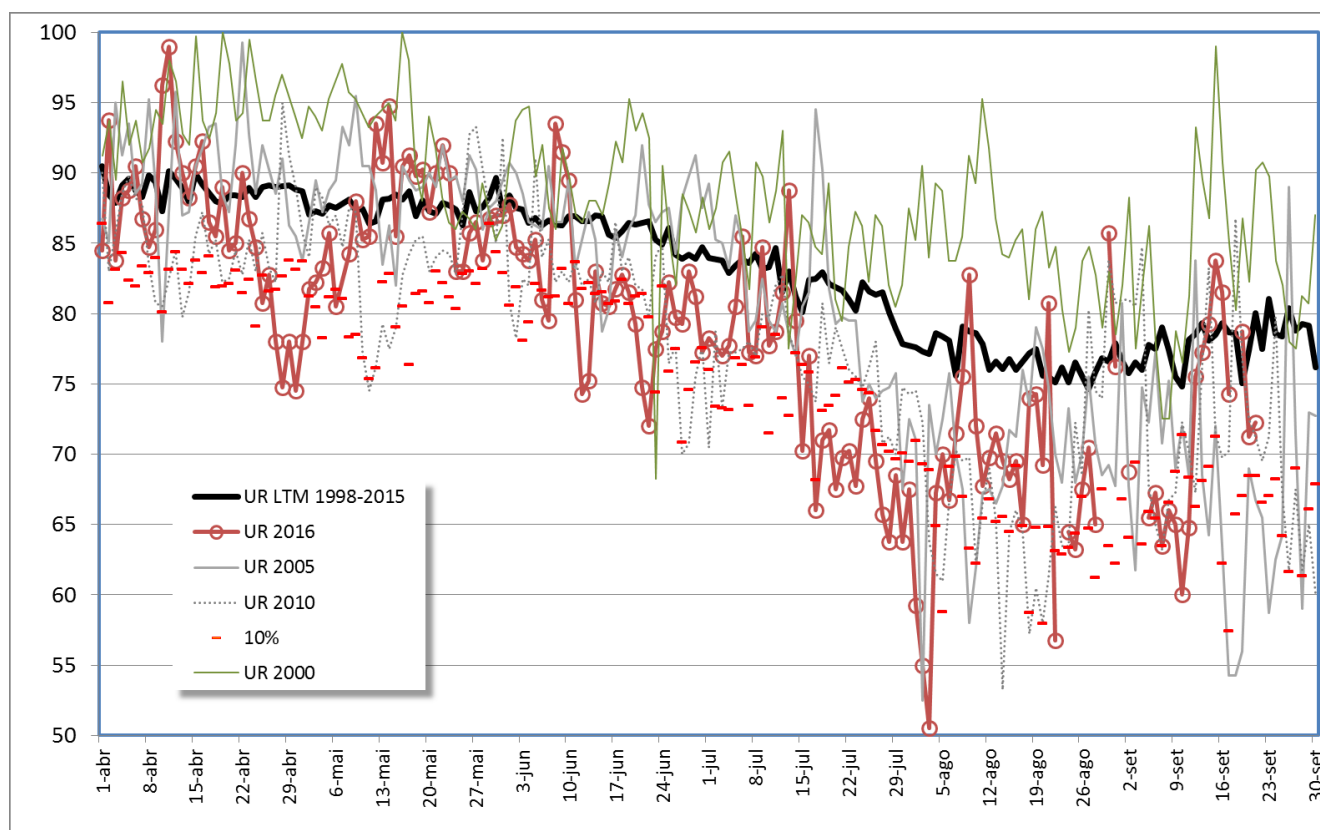
Figura 10. Evolução temporal da umidade relativa do ar (UR) na estação meteorológica de Rio Branco-AC. Atualizada em: 21-Setembro-2016. Fonte dos dados: Instituto Nacional de Meteorologia (INMET).
