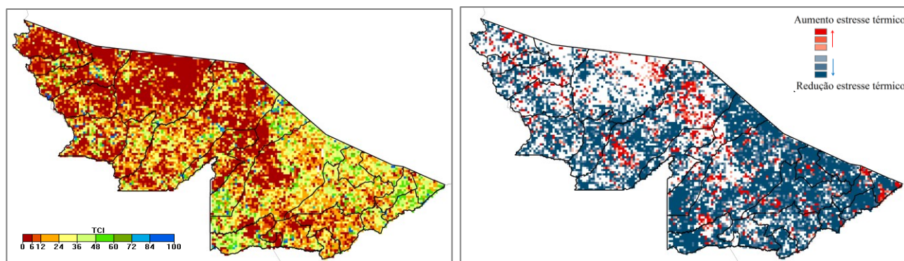
Figura 10. Índice de Condição Térmica da Vegetação (ICT) entre o período de 26 de agosto a 01 de setembro de 2016 (esquerda) e alteração do índice ICT em relação ao período de 10 a 15 de setembro (direita).
