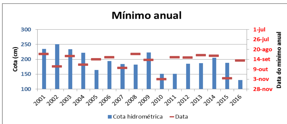
Figura 5. Cotas mínimas anuais registradas no Rio Acre (seção de controle ANA 13600002), segundo o monitoramento da CPRM/ANA (Convencional + Telemétricas), e leituras realizadas pela Defesa Civil (desde Julho de 2016).
