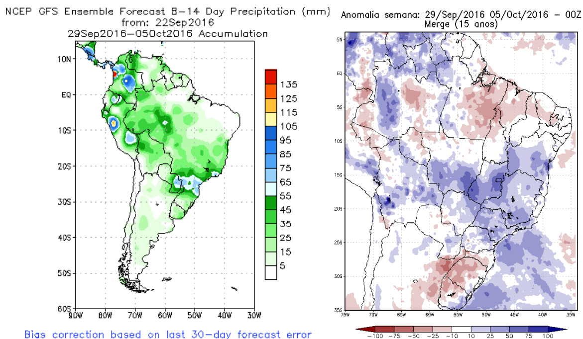
Figura 15. Esq.: Previsão de precipitação no período 29 de setembro a 05 de outubro de 2016, pelo modelo de previsão por conjuntos do Global Forecast System do NCEP/NOAA/EUA. Inicialização em 22 de setembro de 2016. Dir.: Previsão de anomalia de precipitação no período 29 de setembro a 05 de outubro de 2016, pelo modelo de previsão por conjuntos do CPTEC/INPE. Inicialização em 22 de setembro de 2016.
