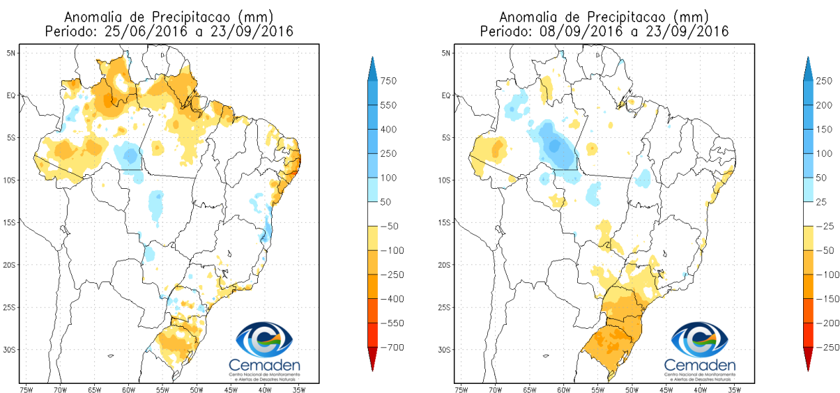
Figura 1. Esq. Anomalia de precipitação média nos últimos 90 dias. Dir. Anomalia de precipitação média nos últimos 15 dias. Atualizada em: 23-Setembro-2016.
