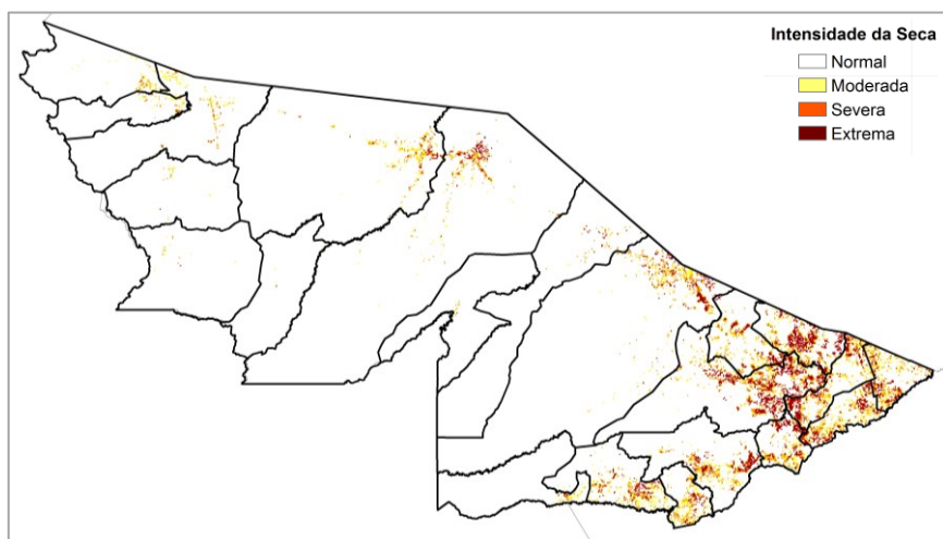
Figura 11. Índice de suprimento de água para a vegetação (VSWI) até 12 de setembro de 2016.
