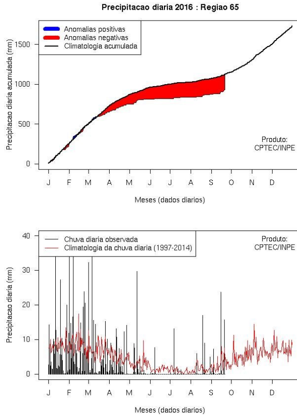
Figura 2. Precipitação acumulada diariamente na região de Rio Branco. FONTE: Centro de Previsão de Tempo e Estudos Climáticos (CPTec/INPE/MCTIC). Atualizada em: 23-Setembro-2016.
