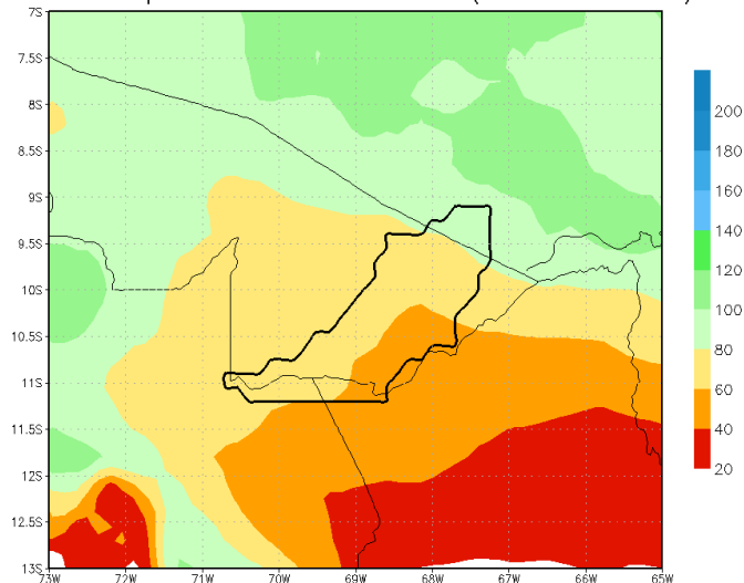
Precipitacao acumulada em 10 dias (mm) : Bacia Rio Acre Previsao a partir de 20160922 00 UTC (media 7 membros)
