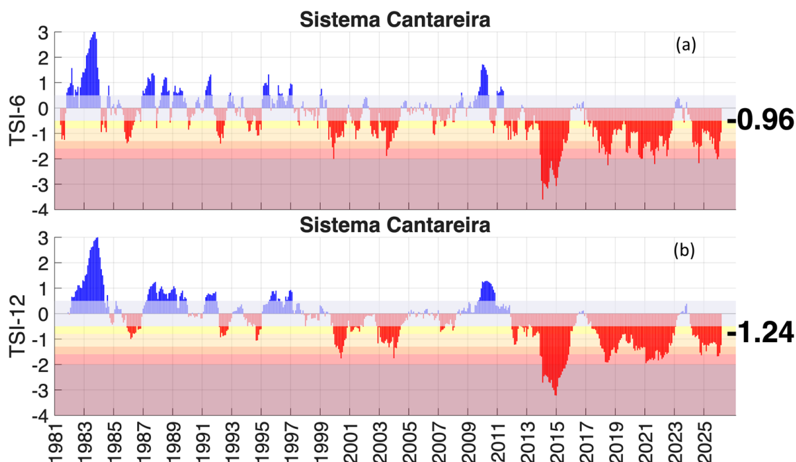
Figura 3. Índice de Seca Bivariado Precipitação-Vazão (TSI) para o Sistema Cantareira, nas escalas temporais de 6 (a) e 12 (b) meses, entre janeiro de 1981 a março de 2026. As faixas coloridas indicam as categorias de seca hidrológica variando entre fraca à excepcional, na seguinte ordem: amarelo (fraca); bege (moderada); laranja (severa); vermelho (extrema) e bordô (excepcional).
