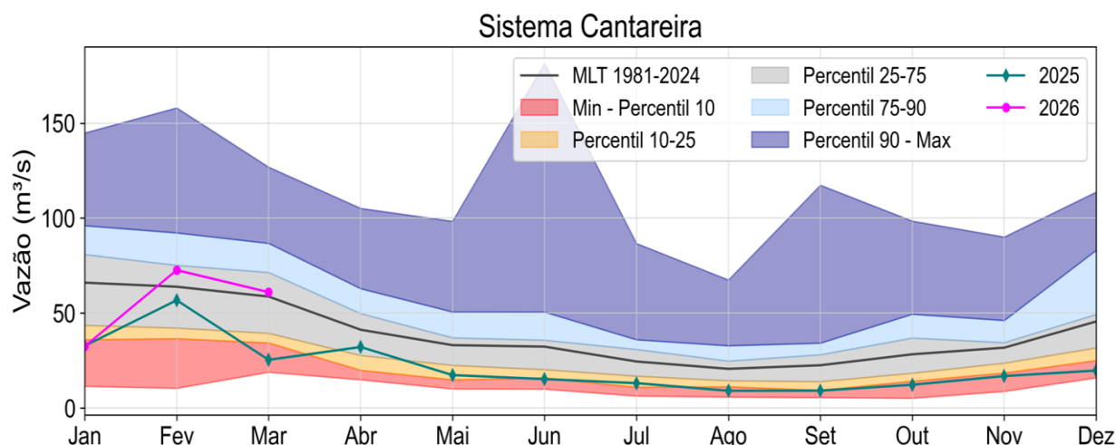
Figura 2. Vazão afluyente à bacia do Sistema Cantareira (Sistema Equivalente + Paiva Castro), em m^3/s , no período de janeiro a março de 2026 (linha magenta). As linhas preta e verde representam, respectivamente, a vazão média mensal histórica (1981–2024) e a vazão observada em 2025. As vazões mínimas e máximas do histórico estão indicadas pelas faixas em vermelho e azul escuro. Fonte dos dados: SABESP.
