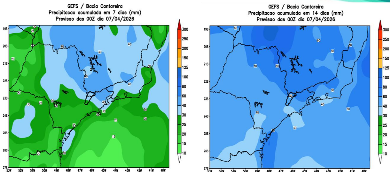
Figura 5. Previsão de precipitação acumulada em milímetros (mm) nos próximos 7 (a) e 14 (b) dias para a bacia de captação do Sistema Cantareira, segundo a previsão do modelo numérico GENS/NOAA. A área da bacia de captação do Sistema Cantareira é indicada no centro da figura com linha preta espessa.
