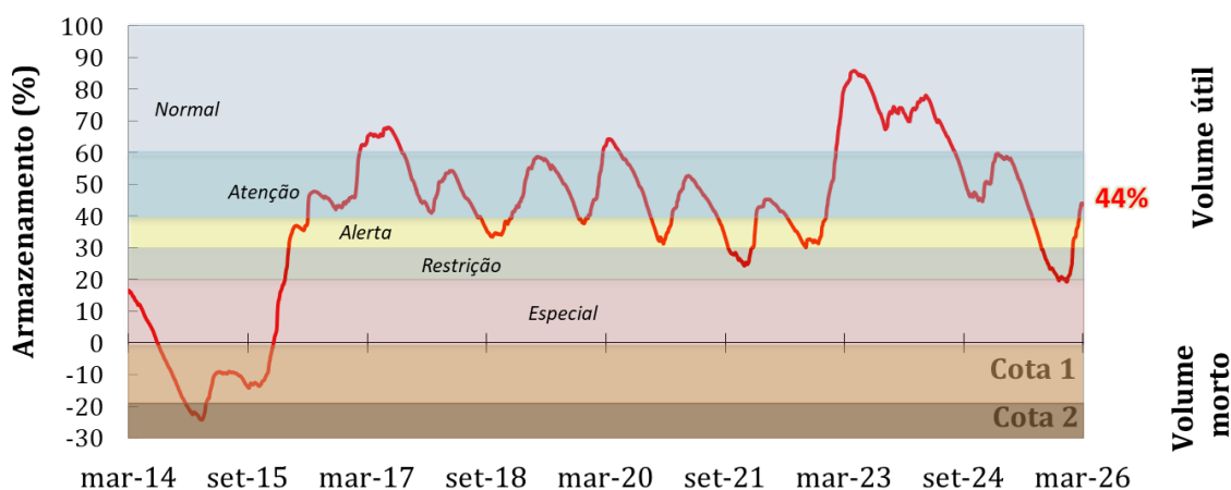
Figura 4. Evolução diária do armazenamento (%) do Sistema Cantareira entre 01 de março de 2014 e 28 de março de 2026. Fonte de dados: SABESP. Área marrom claro corresponde à primeira cota do volume morto (182,5 hm 3 ) e marrom escuro à segunda cota do volume morto (105 hm 3 ). As faixas coloridas referem-se às faixas de operação de acordo com a resolução conjunta da ANA/DAEE Nº 925/2017, com volume útil de 982 hm 3 .
