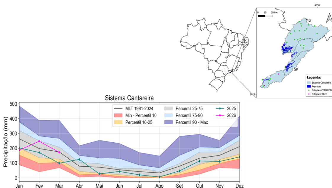
Figura 1: Precipitação mensal na bacia do Sistema Cantareira, em mm, de acordo com os dados do CEMADEN, entre janeiro e março de 2026 (linha magenta). Ano hidrológico: outubro – setembro. As linhas preta e verde representam, respectivamente, a precipitação média mensal histórica (1981–2024) e a precipitação observada em 2025. As precipitações mínimas e máximas do histórico estão indicadas pelas faixas em vermelho e azul escuro. Os pluviômetros operantes atualmente: 26 do CEMADEN (pontos verdes) e 7 do DAEE/ SAISP (pontos magentas).
