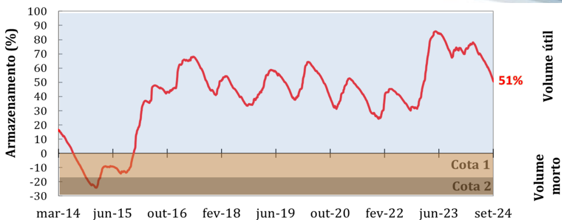
Figura 5. Evolução diária do nível de armazenamento (%) do Sistema Cantareira entre o período de março de 2014 a setembro de 2024. Área em azul corresponde ao volume útil do reservatório (982 hm 3 ), em marrom claro à primeira cota do volume morto (182,5 hm 3 ) e em marrom escuro à segunda cota do volume morto (105 hm 3 ). Fonte dos dados: SABESP.
