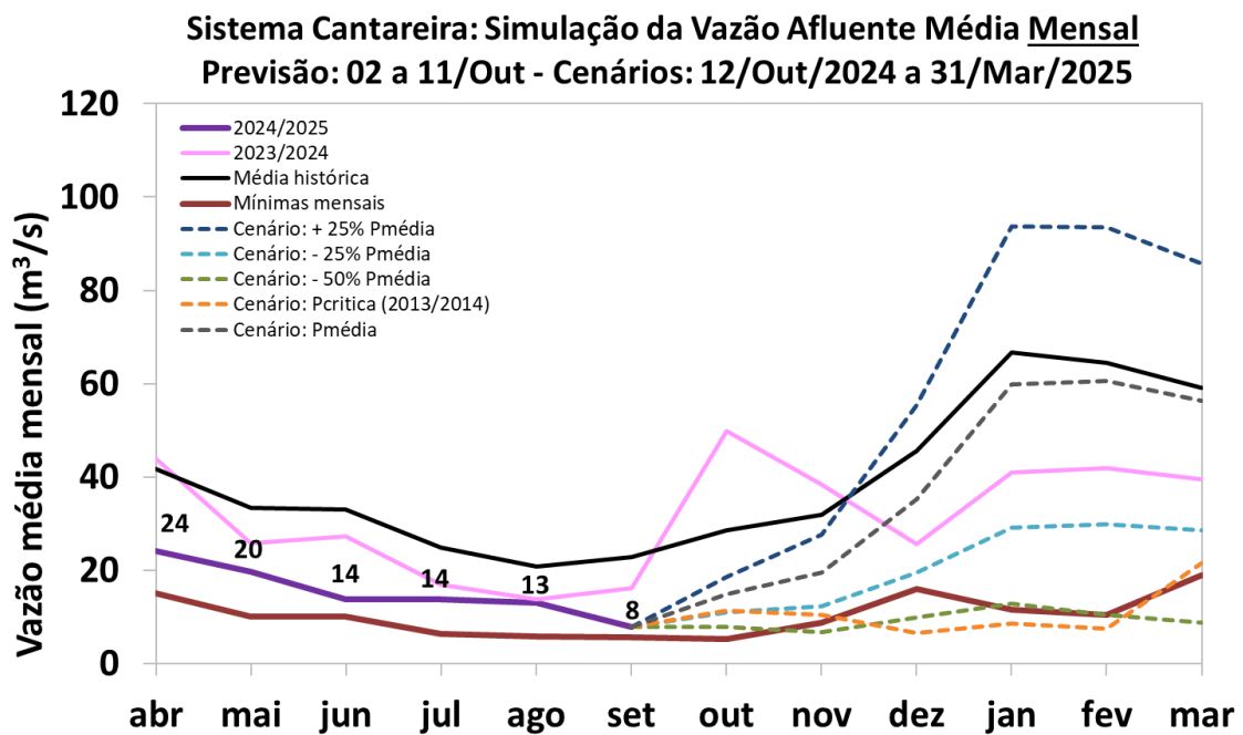
Figura 10. Histórico (linhas contínuas) e simulação de vazão média mensal (em m 3 /s) afluyente ao Sistema Cantareira (linhas tracejadas) considerando a previsão e cinco cenários de precipitação: 50% (verde) e 25% abaixo da média histórica (azul claro); na média histórica (cinza) e 25% acima da média histórica (azul escuro) e cenário crítico (laranja). As linhas espessas representam as vazões médias mensais observadas, de acordo com a SABESP: média histórica (preto); mínimos mensais (marrom); série de abril de 2023 a março de 2024 (magenta); e série de abril a setembro de 2024 (roxo).
