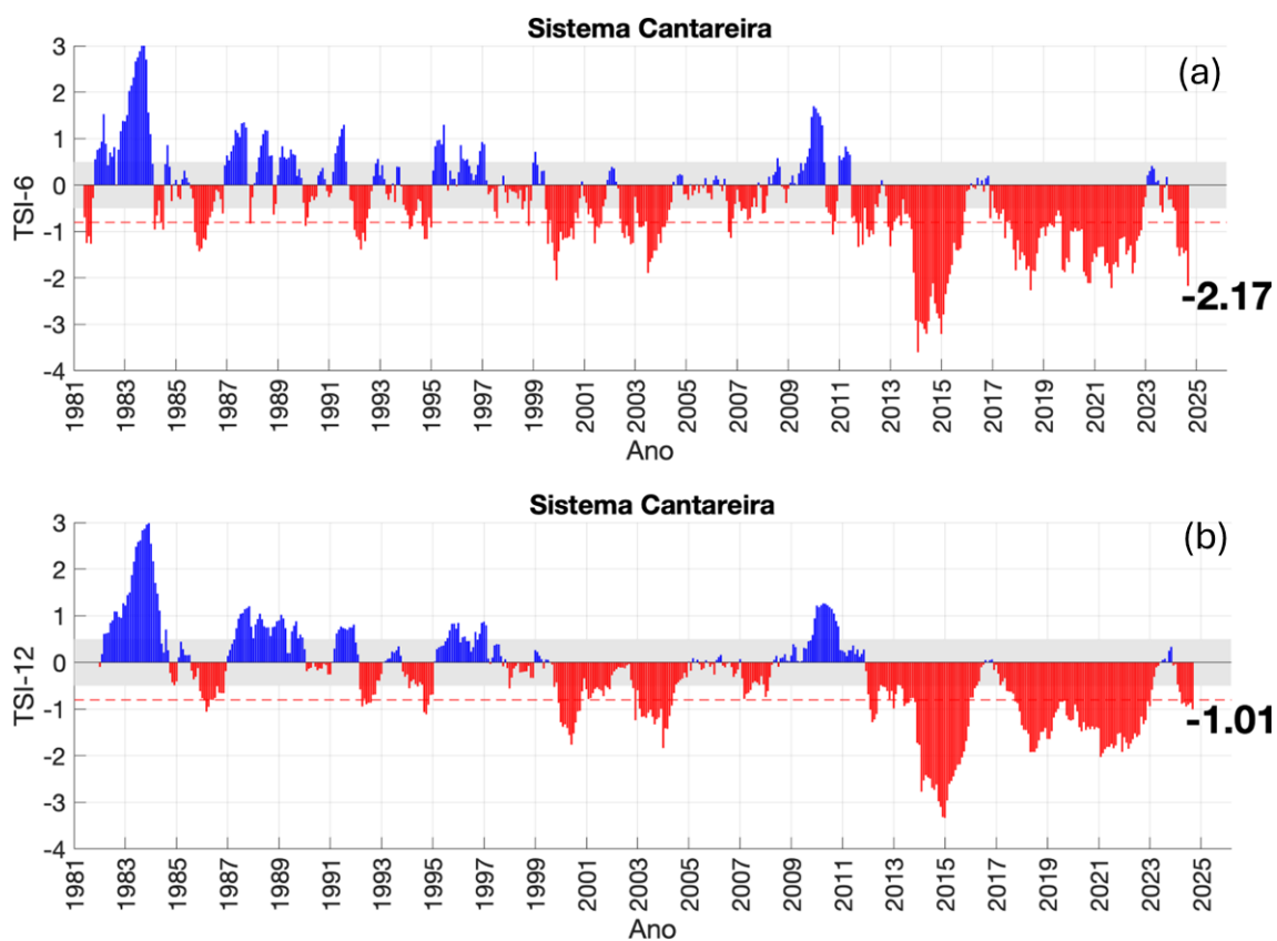
Figura 3. Índice Padronizado Bivariado Precipitação-Vazão (TSI) para o Sistema Cantareira, nas escalas temporais de 6 (a) e 12 (b) meses, entre janeiro de 1981 a setembro de 2024. A linha vermelha pontilhada indica o limiar entre uma condição de seca hidrológica fraca e moderada à excepcional.
