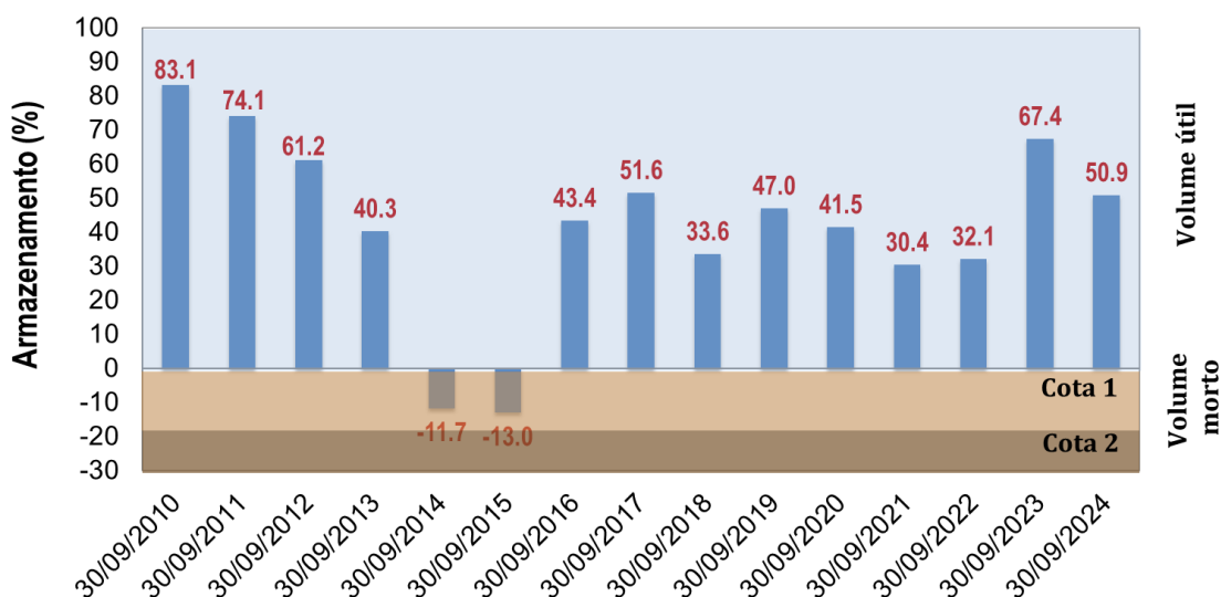
Figura 6. Evolução do volume armazenado (%) nos reservatórios do Sistema Cantareira para o final do mês de setembro, entre os anos de 2010 e 2024.
