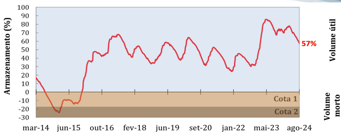
Figura 5. Evolução diária do nível de armazenamento (%) do Sistema Cantareira entre o período de março de 2014 a agosto de 2024. Área em azul corresponde ao volume útil do reservatório (982 hm 3 ), em marrom claro à primeira cota do volume morto (182,5 hm 3 ) e em marrom escuro à segunda cota do volume morto (105 hm 3 ). Fonte dos dados: SABESP.
