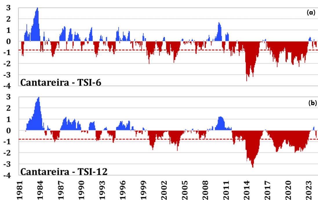
Figura 3. Índice Padronizado Bivariado Precipitação-Vazão (TSI) para o Sistema Cantareira, nas escalas temporais de 6 e 12 meses, entre janeiro de 1981 a março de 2024. A linha vermelha pontilhada indica o limiar entre uma condição de seca hidrológica fraca e moderada à excepcional.
