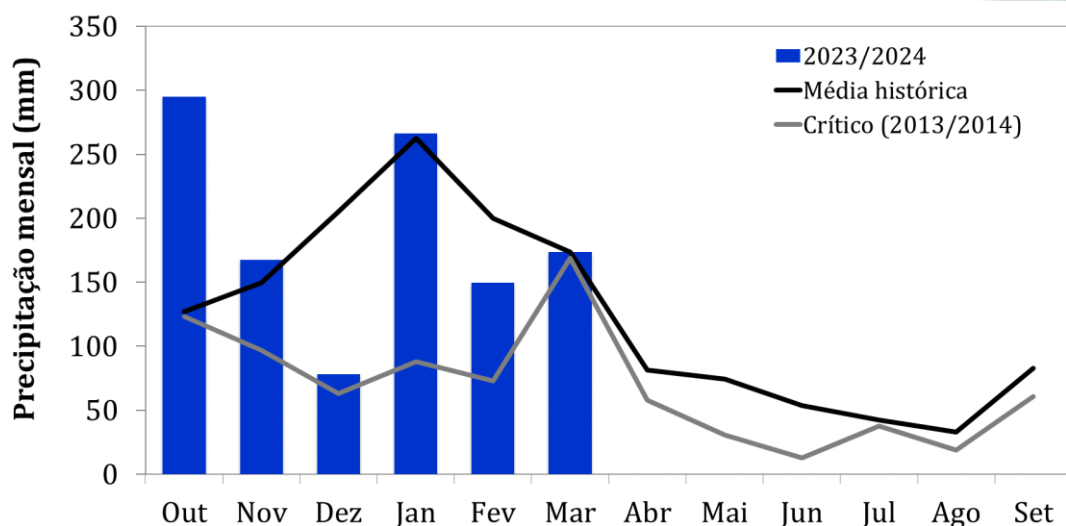
Figura 2. Precipitação mensal na bacia do Sistema Cantareira, em mm, de acordo com os dados do CEMADEN, entre outubro de 2023 e março de 2024 (barras em azul). Ano hidrológico: outubro – setembro. As linhas em preto e cinza representam, respectivamente, a precipitação média histórica (1983-2023) e a precipitação crítica do histórico, compreendida entre outubro de 2013 a setembro de 2014.
