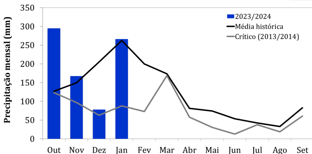
Figura 2. Precipitação mensal na bacia do Sistema Cantareira, em mm, de acordo com os dados do CEMADEN, entre outubro de 2023 e janeiro de 2024 (barras em azul). Ano hidrológico: outubro – setembro. As linhas em preto e cinza representam, respectivamente, a precipitação média histórica (1983-2023) e a precipitação crítica do histórico, compreendida entre outubro de 2013 a setembro de 2014.
