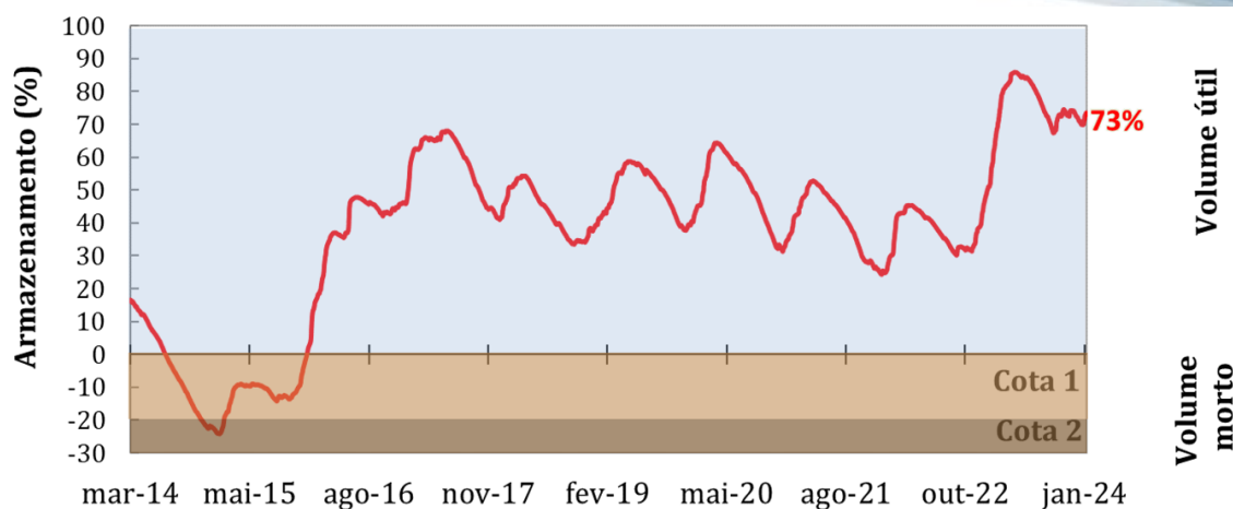
Figura 5. Evolução diária do nível de armazenamento (%) do Sistema Cantareira entre o período de março de 2014 a janeiro de 2024. Área em azul corresponde ao volume útil do reservatório (982 hm 3 ), em marrom claro à primeira cota do volume morto (182,5 hm 3 ) e em marrom escuro à segunda cota do volume morto (105 hm 3 ). Fonte dos dados: SABESP.
