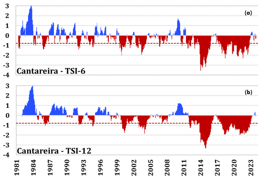
Figura 3. Índice Padronizado Bivariado Precipitação-Vazão (TSI) para o Sistema Cantareira, nas escalas temporais de 6 e 12 meses, entre janeiro de 1981 a janeiro de 2024. A linha vermelha pontilhada indica o limiar entre uma condição de seca hidrológica fraca e moderada à excepcional.
