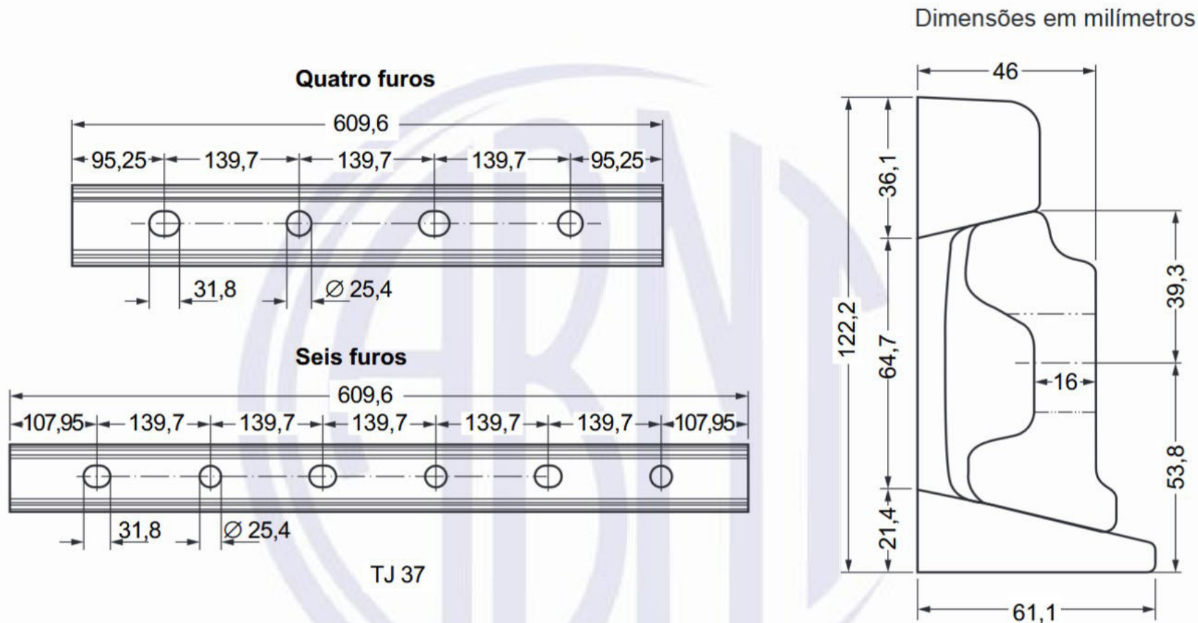
Figura A.1 – Dimensões da tala de junção TJ 37
