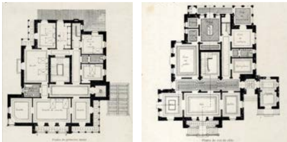
Figura 12 – Planta do primeiro e segundo piso da Quinta dos Lagos, Sintra. Arq. Francisco Carlos Parente, 1906. Fonte: Architectura Portuguesa , Lisboa, ano 1, n. 3, 1908.
