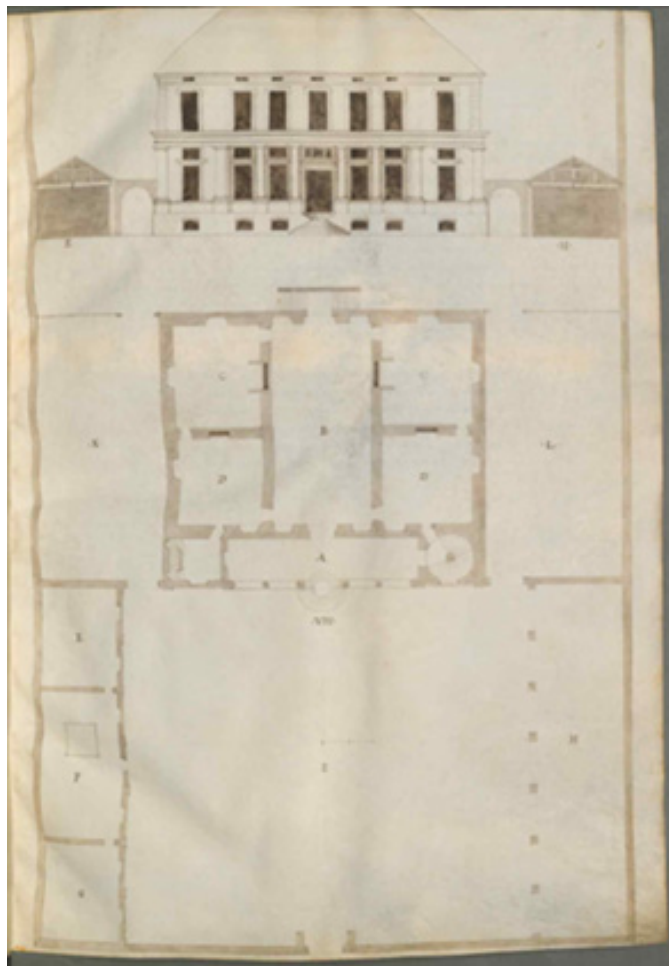
Figura 14 – Planta baixa e elevação da residência de uma villa , presentes no sexto livro do tratado de Serlio. Fonte: Serlio (1618, p. 5).
