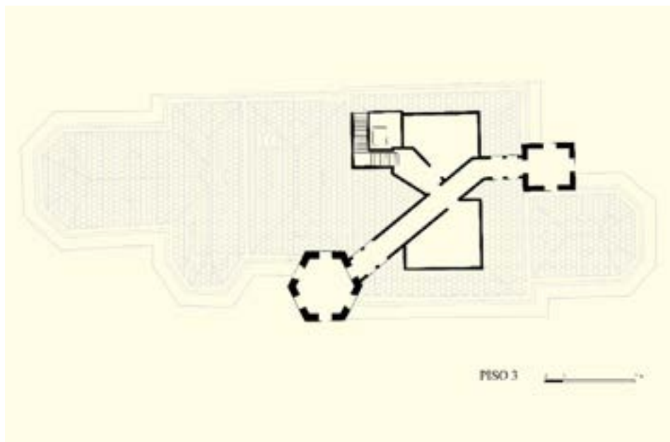
Figura 15 – Planta do sótão. Fonte: Acervo da Administração Hidroviária da Amazônia Oriental, atual órgão que ocupa o Palacete Bibi Costa. Deste acervo, retirou-se o levantamento realizado pelo DPJ, escritório de arquitetura de Belém. Adaptada por Beatriz Maneschy, 2019.
