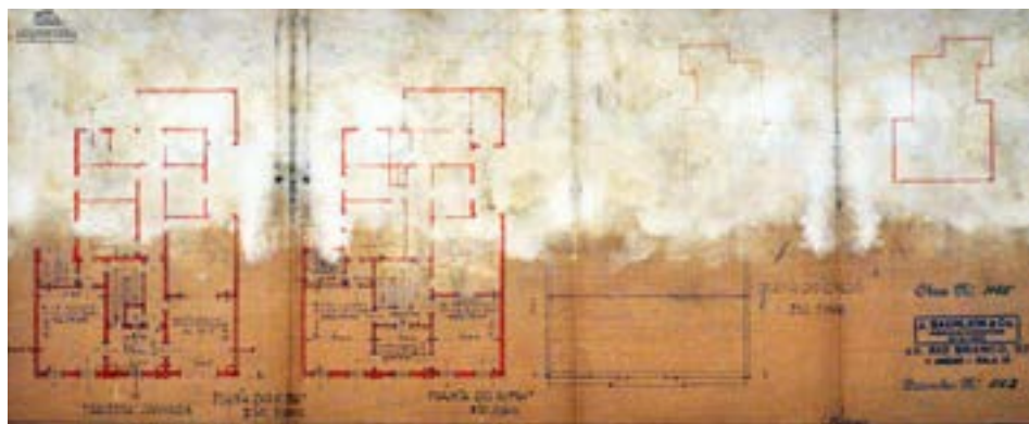
Figura 5 – Plantas baixas e implantação da casa nº 18 – processo nº 18.401/27. Fonte: AGCRJ.
