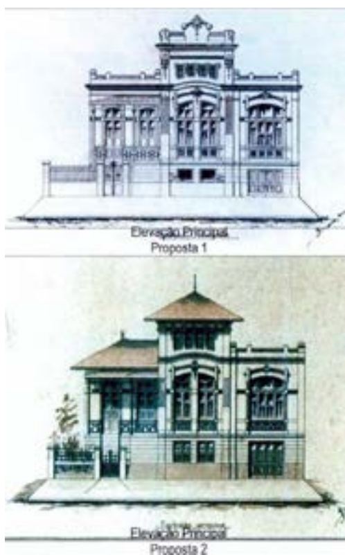
Figura 5 – Fachadas desenhadas por José Sidrim para o projeto do Palacete Orlando Lima. Fonte: Ecletismo na arquitetura residencial de José Sidrim , p. 186.
