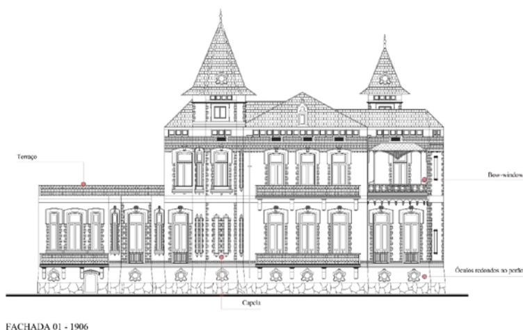
Figura 6 – Elevação da fachada onde atualmente localiza-se a rua Joaquim Nabuco. Fonte: Acervo da Administração Hidroviária da Amazônia Oriental, atual órgão que ocupa o Palacete Bibi Costa. Deste acervo, retirou-se o levantamento realizado pelo DPJ, escritório de arquitetura de Belém. Adaptada por Beatriz Maneschy, 2019.
