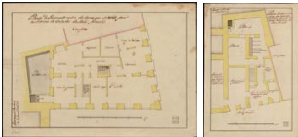
Figura 10 – Plantas do piso térreo e piso nobre das casas que se hande fazer no extremo da Calçada da Rua da Formosa. Fonte: Marquês de Pombal, 12 de Janeiro 1772.
