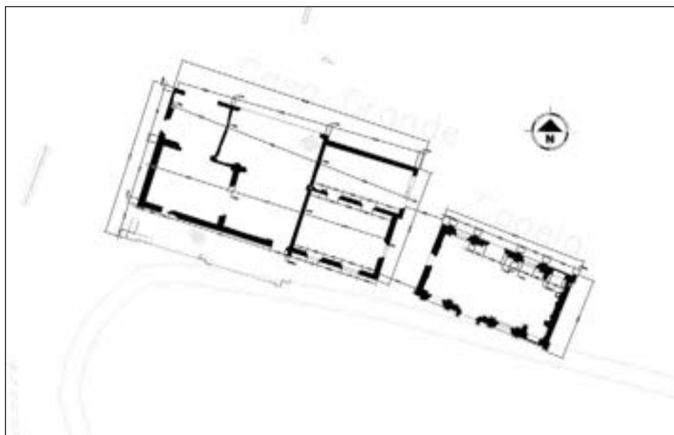
Figura 5 – Plantas baixas da casa senhorial e da capela do engenho Murutucu. Desenho em CAD. Fonte: Acervo pessoal de Fernando Marques. Adaptada.
