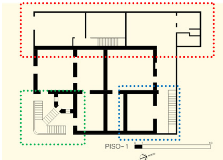
Figura 13 – Em vermelho está destacada a localização do anexo construído entre 2004 e 2006; em verde, o antigo acesso social; e em azul, o antigo acesso de serviço. Fonte: levantamento realizado por DPJ em 2014-2017 e adaptado por Caroline M. F. Rodrigues e Ailla C. de C. Raiol, 2018.
