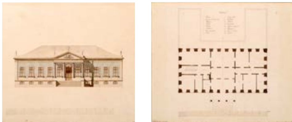
Figura 8 – Palacete neoclássico: alçado e planta do piso nobre. José Luis Monteiro, [Assin.] Terminado a 4 de Novembro de 1865. Tinta-da-china e aguarela polícroma sobre papel. Fonte: Arquivo Histórico da Câmara Municipal de Lisboa (AHCML) - JLM-DA - 01.3/1 e /2/3/4/5.
