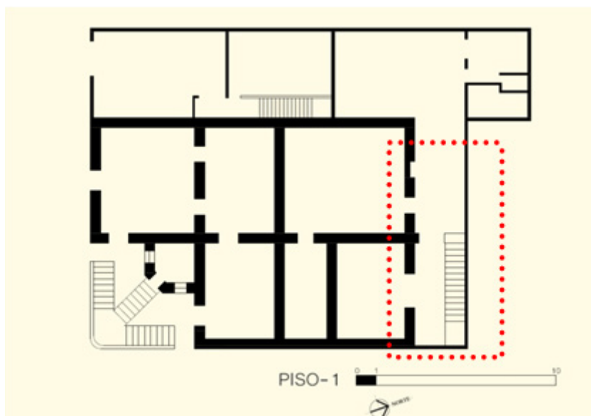
Figura 8 – Antiga localização da escada no pavimento térreo. Fonte: levantamento realizado por DPJ em 2014-2017 e adaptado por Caroline M. F. Rodrigues e Ailla C. de C. Raiol, 2018.
