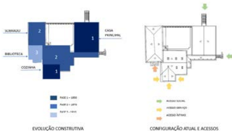
Figura 4 – Planta baixa com esquemas hipotéticos sobre a evolução construtiva da casa. Fonte: a autora (2019).
