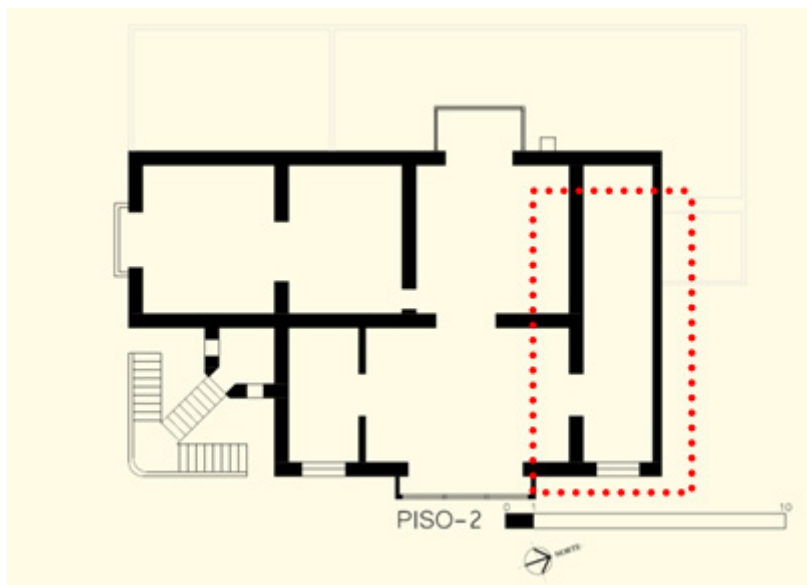
Figura 9 – Antiga localização da escada no primeiro pavimento. Fonte: levantamento realizado por DPJ em 2014-2017 e adaptado por Caroline M. F. Rodrigues e Ailla C. de C. Raiol, 2018.
