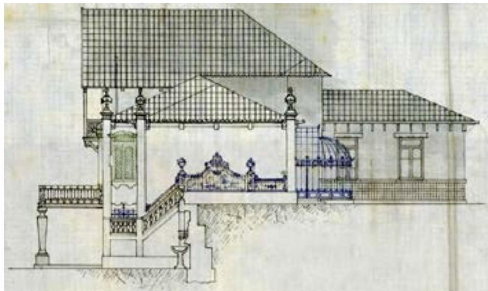
Figura 6 – Projeto de 1910, alçado nascente. Fonte: Arquivo Histórico Municipal do Porto.
