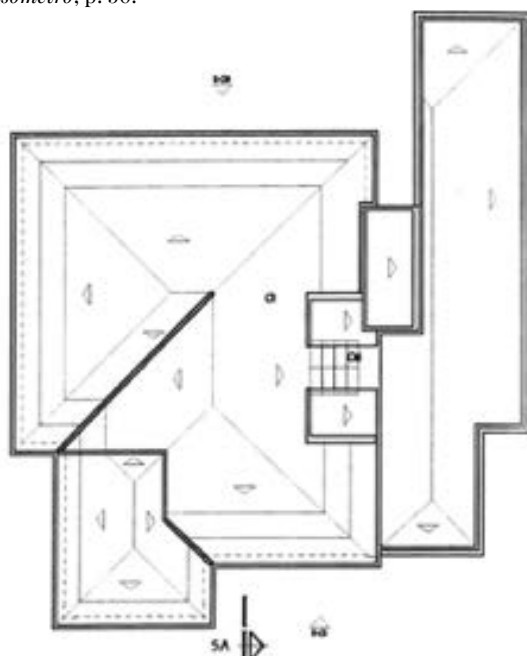
Figura 12 – Planta de cobertura edifício geminado Parque da Residência. Fonte: Parque da Residência e Estação Gasômetro , p. 50. 5
