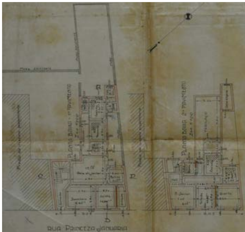
Figura 7 – Plantas baixas da casa de nº 16. s.d. Fonte: AGCRJ.
