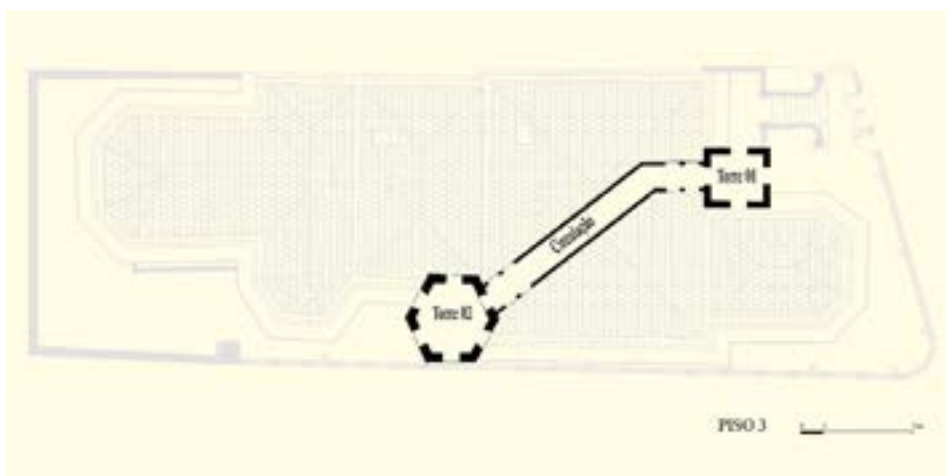
Figura 12 – Planta baixa do sótão, nota-se o fechamento do terraço com o telhado, quando foi prolongado o segundo pavimento e a circulação entre as duas torres. Fonte: Acervo da Administração Hidroviária da Amazônia Oriental, atual órgão que ocupa o Palacete Bibi Costa. Deste acervo, retirou-se o levantamento realizado pelo DPJ, escritório de arquitetura de Belém. Adaptada por Beatriz Maneschy, 2019.
