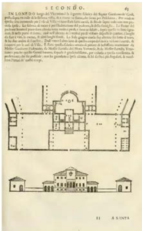
Figura 13 – Villa Godi , em Vicenza, Itália. Planta baixa e elevação. Fonte: Palladio (1616, p. 65).
