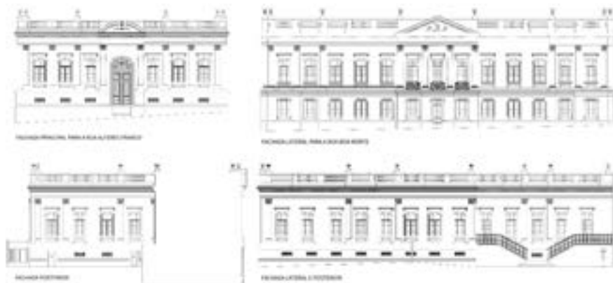
Figura 11 – Fachadas do palacete em seu estado atual. Fonte: elaborada pelas autoras a partir do Projeto de restauração Palacete Levy: memorial de restauro (2005), de Juliana B. P. Scariato. Anexos n. 6,7,8,9, Elevações.
