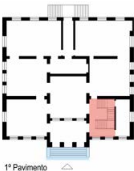
Figura 12 – Planta baixa do Solar do Barão do Guamá, com demarcações da escada de acesso à edificação (em azul) e escadas de circulação vertical interna (em vermelho). Fonte: acervo pessoal de Vithória Silva, 2019.
