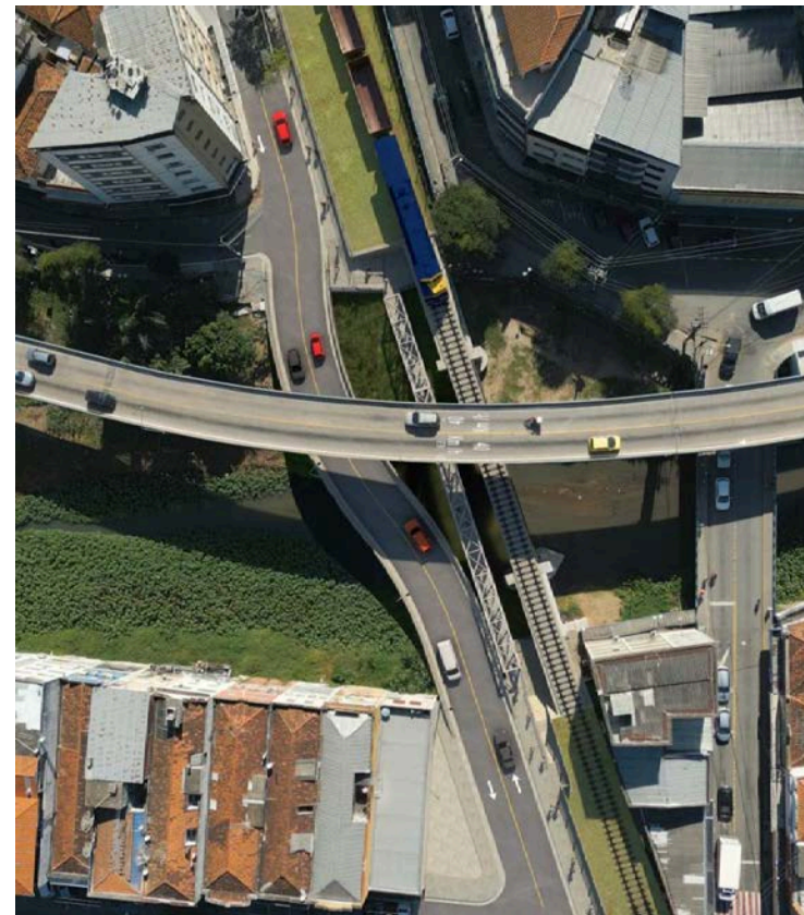
Complexo Viário Barra do Pirai/RJ
