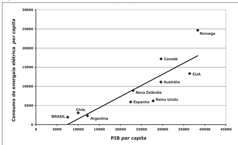
Figura 2.4. Consumo de eletricidade per capita com referência ao PIB, 2004
