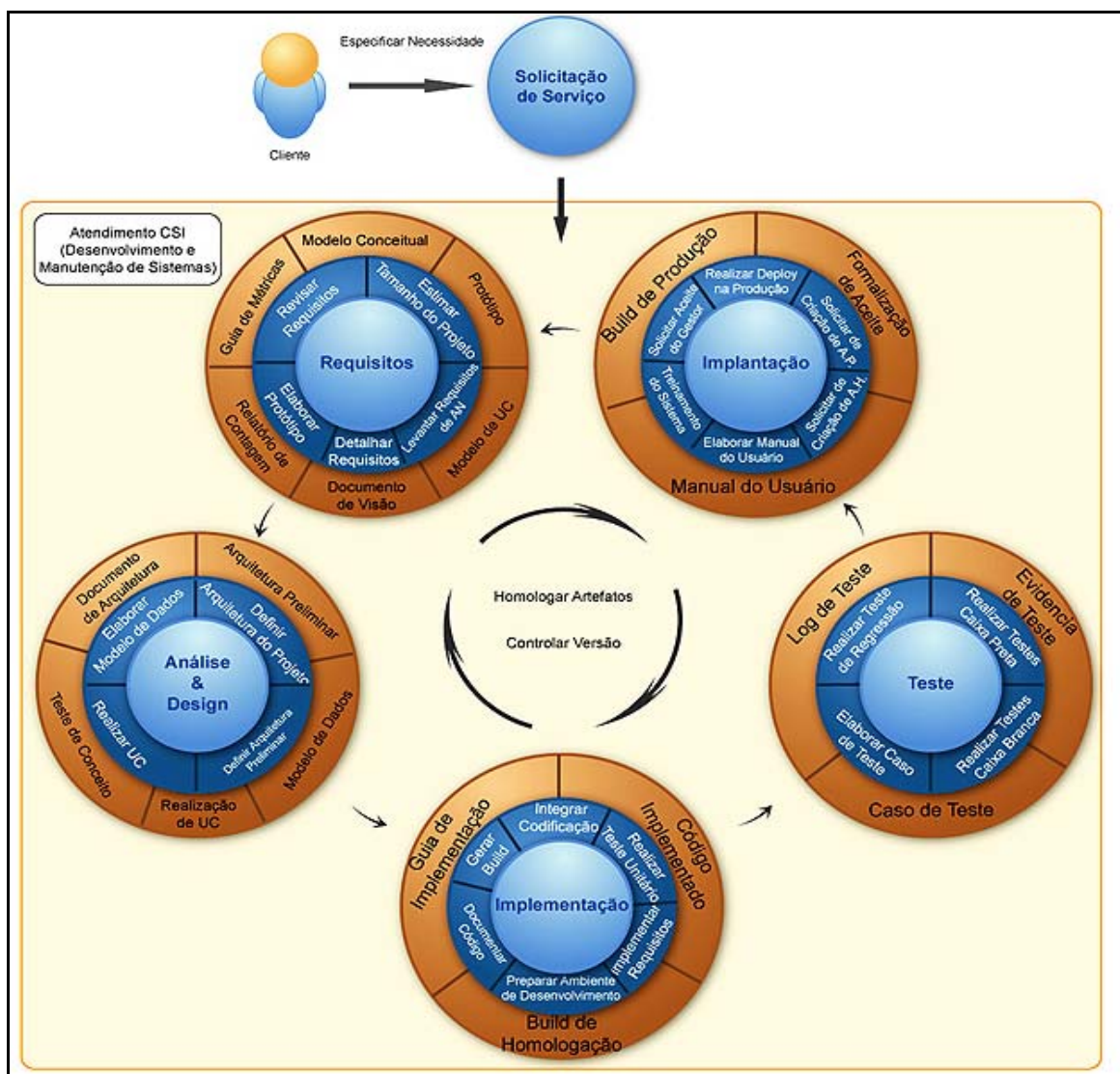
Figura. Fluxo da Metodologia de Desenvolvimento de Sistemas
