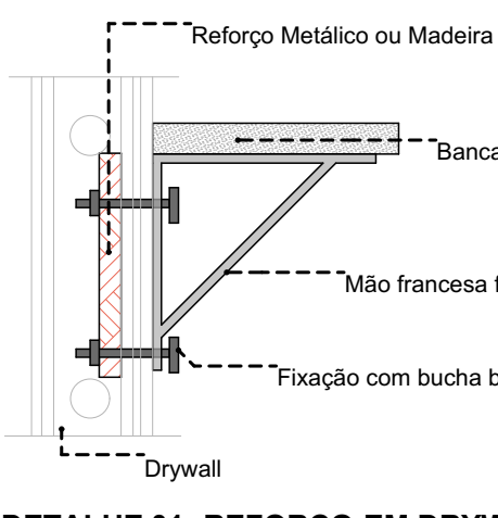
DETALHE 01: REFORÇO EM DRYWALL
