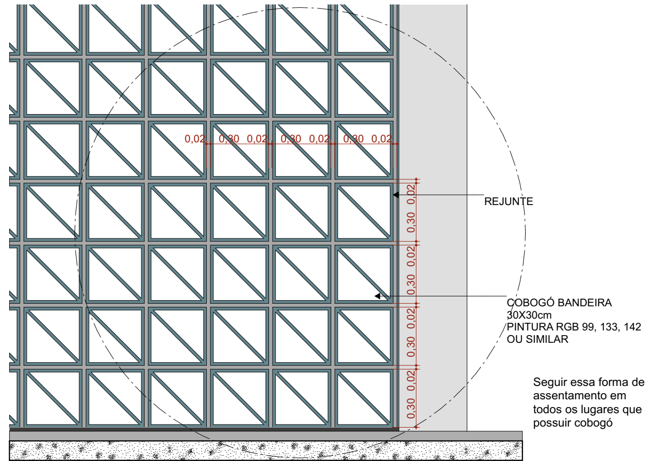
Detalhamento Assentamento Cobogó Escala: 1:20
