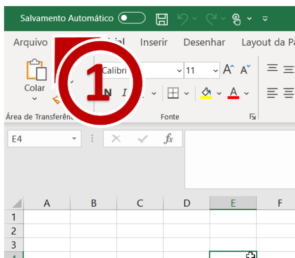
Figura 6 - Menu Arquivo
