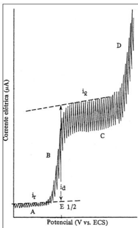
Figura 1- Polarograma de espécie eletroreduzível.
