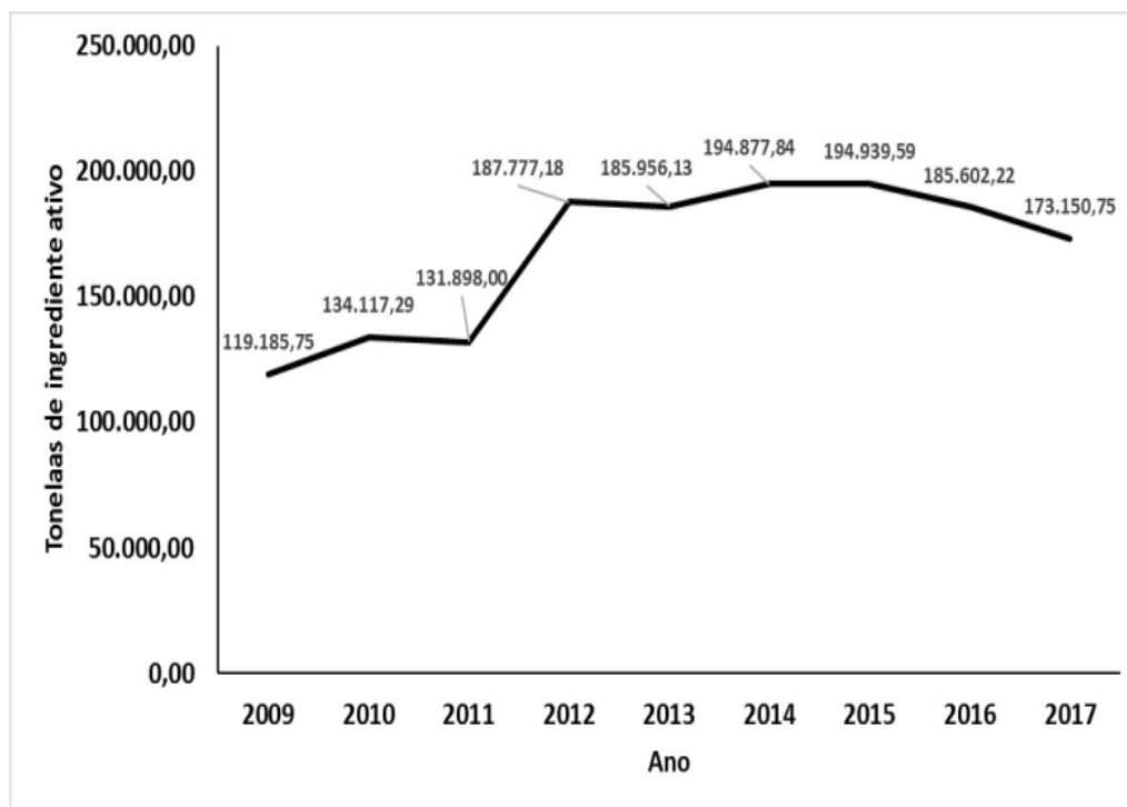
Figura 1. Distribuição anual da quantidade, em toneladas, do ingrediente ativo Glifosato comercializada no Brasil, 2009 a 2017.
