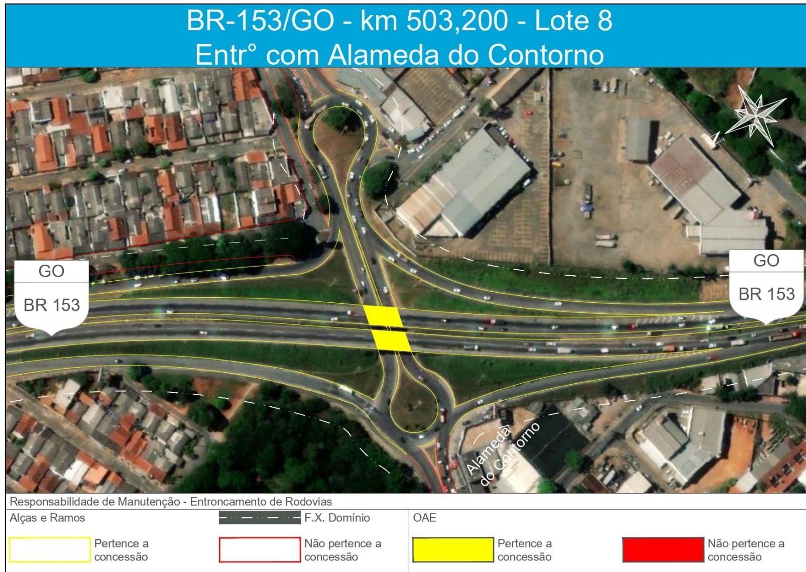
Figura 40 - Interseções BR-153/GO – Entroncamento com a Av. Gonzaga Leite
