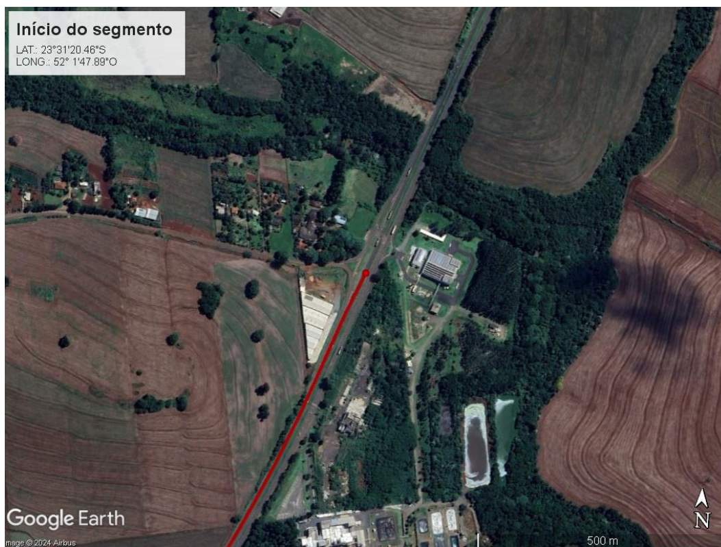
Figura 14 – Início do Segmento da PR-317
