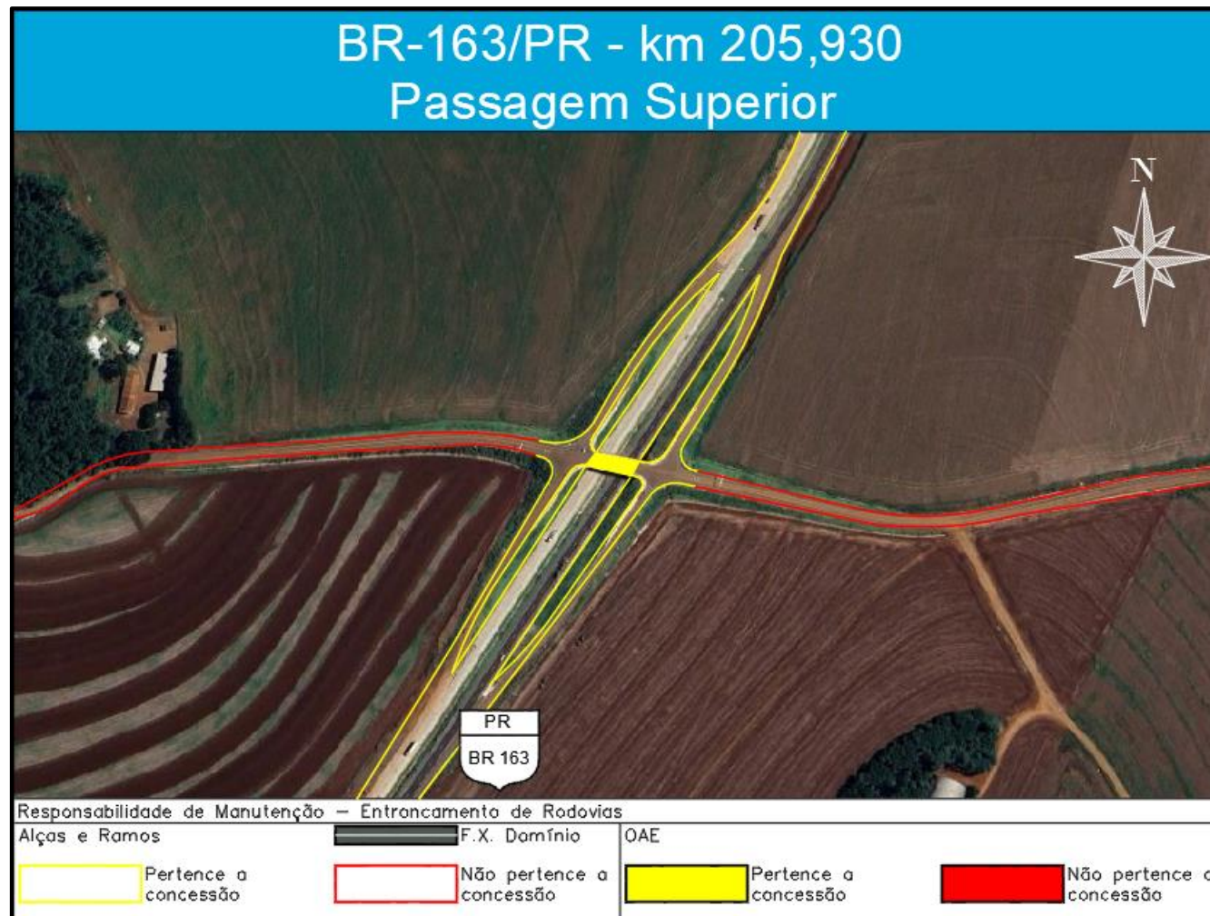
Figura 38 - BR 163/PR km 205,930 Passagem Superior
