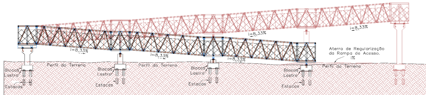
Figura 22 – Croqui Básico Passarela
