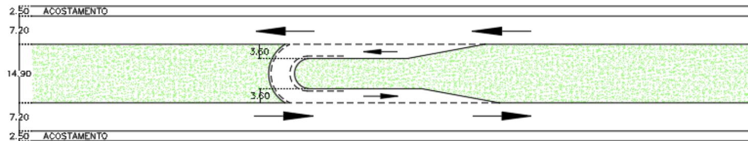
Figura 25 – Croqui Básico Retorno em U
