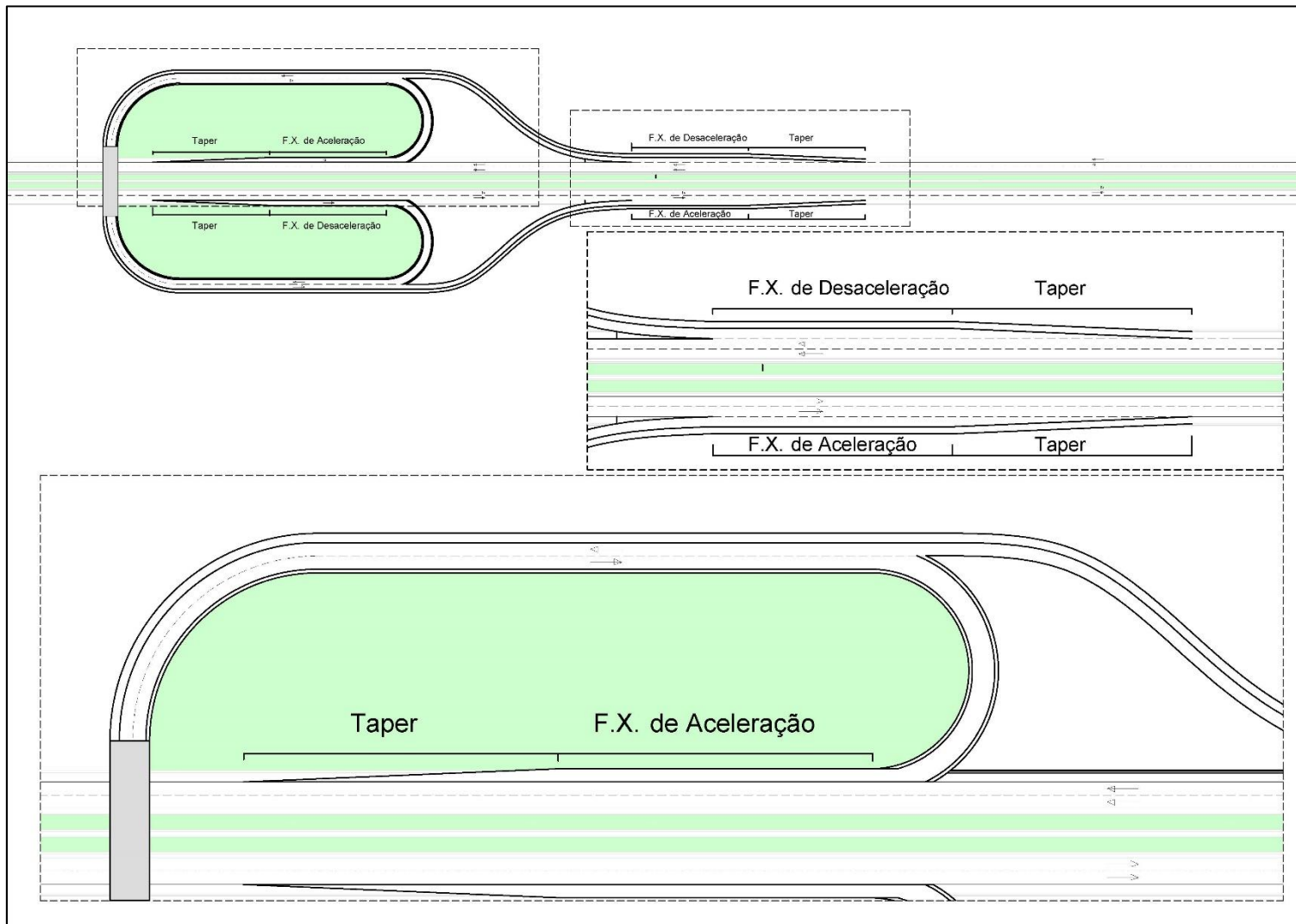
Figura 29 – Croqui Básico Parclo
