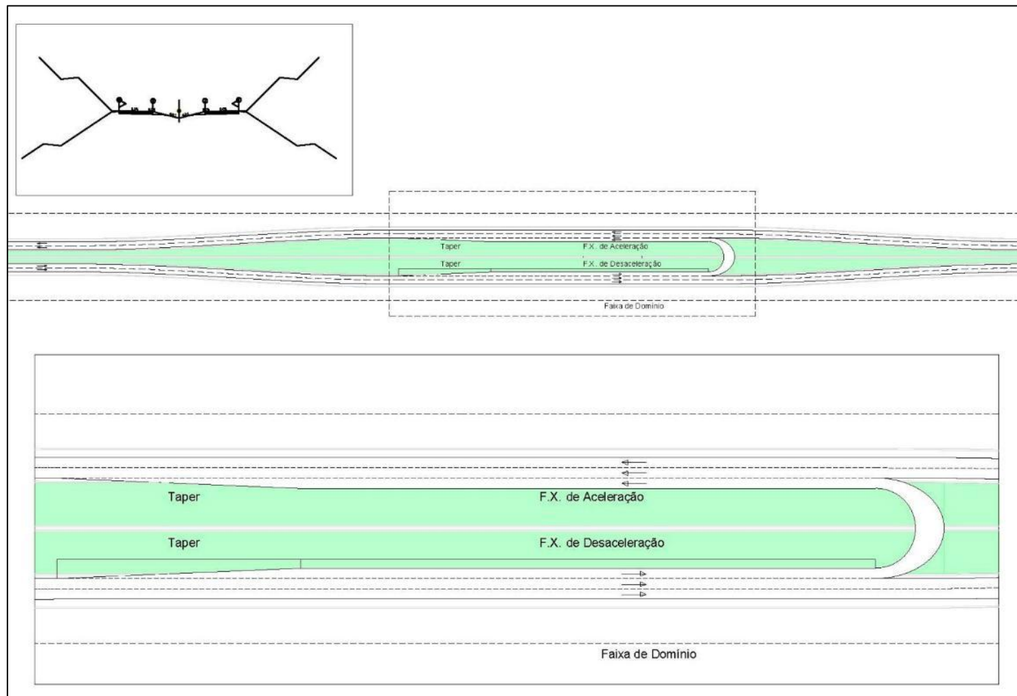
Figura 15 - Croqui Básico de Retorno em U
