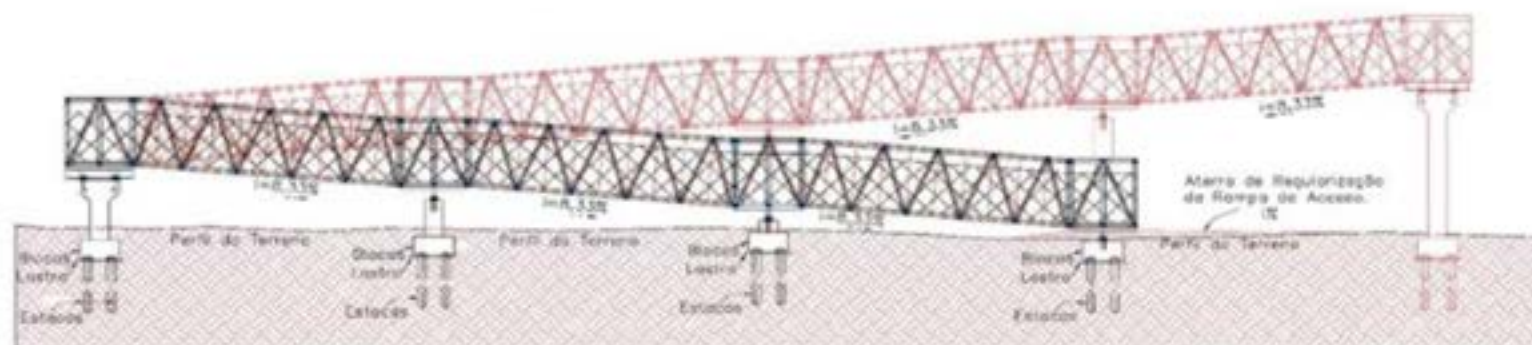
VISTA LONGITUDINAL B-B 1/ ESCALA
