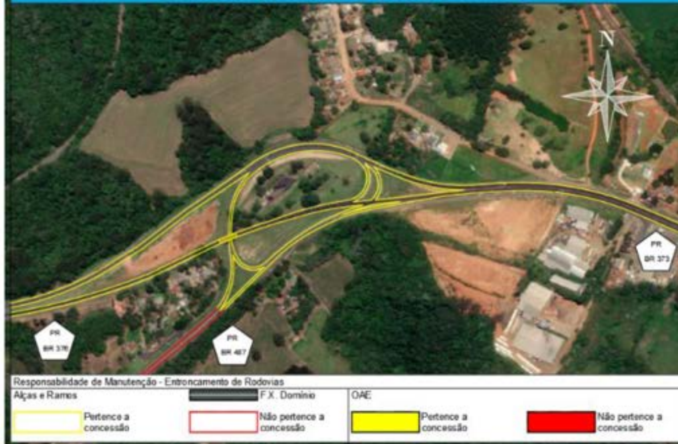
Figura 54 - Interseção na BR-376/PR no km 469,000
