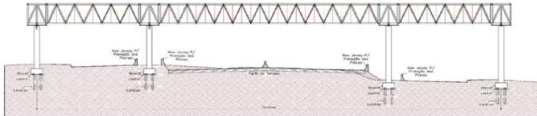
VISTA TRANSVERSAL A-A 1/ ESCALA
