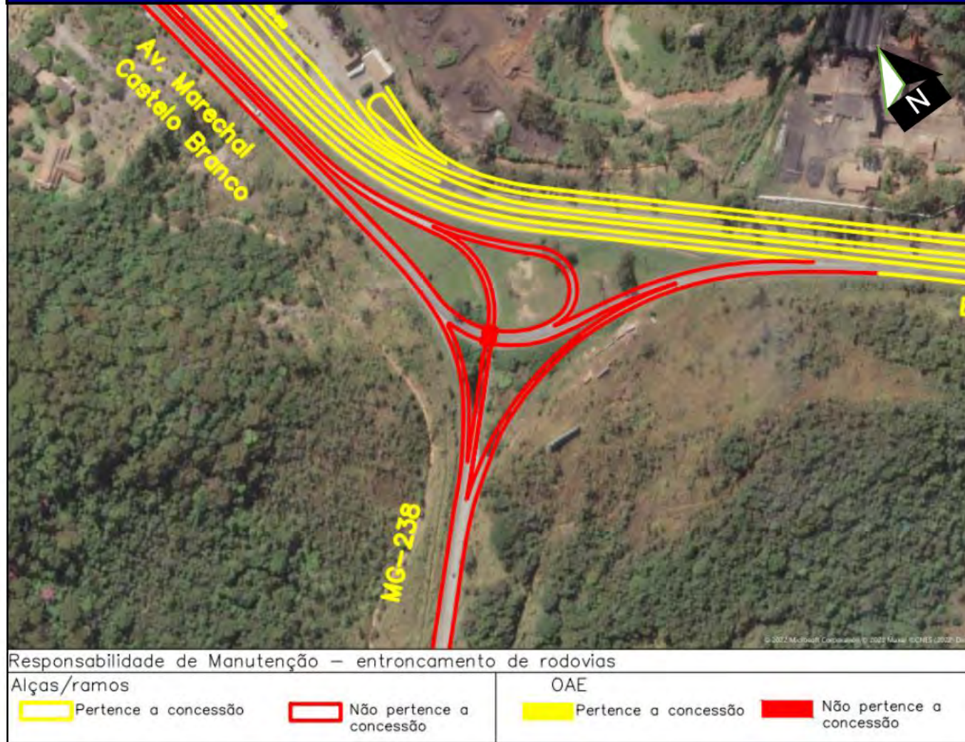
Figura 42 – Interseções BR-040/MG – Entroncamento com Av. Marechal Castelo Branco/MG-238
