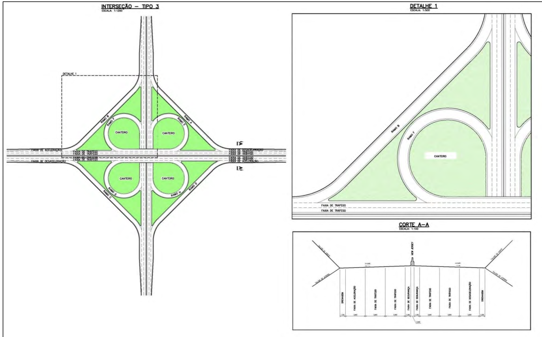
Figura 16 – Croqui Básico Trevo
