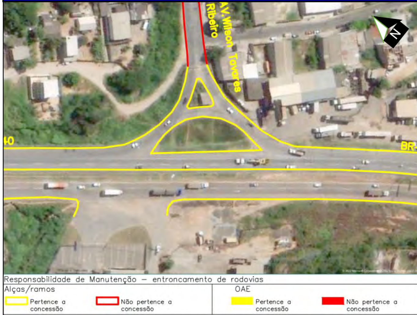
Figura 44 – Interseções BR-040/MG – Entroncamento com Av. Wilson Tavares Ribeiro
