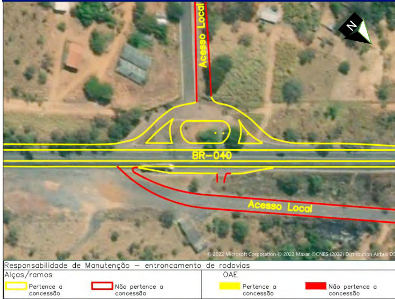
Figura 30 – Interseções BR-040/MG – km 279,000
