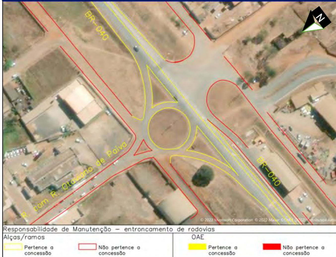
Figura 21 – Interseções BR-040/GO – Entroncamento com R. Otaviano de Paiva/Cristalina
