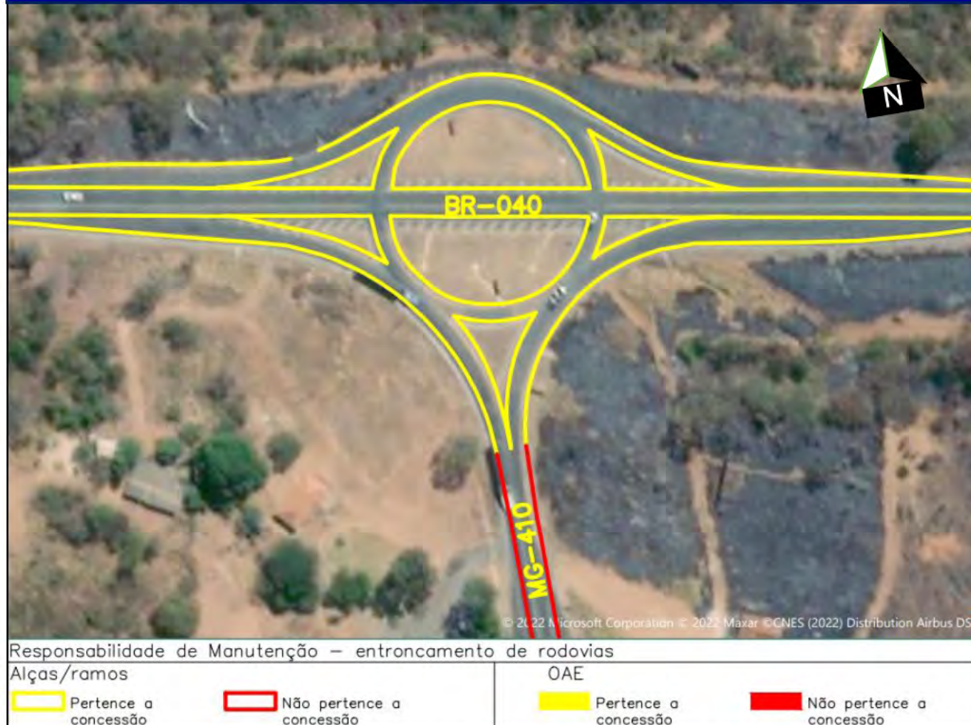
Figura 23 – Interseções BR-040/MG – Entroncamento com MG-410
