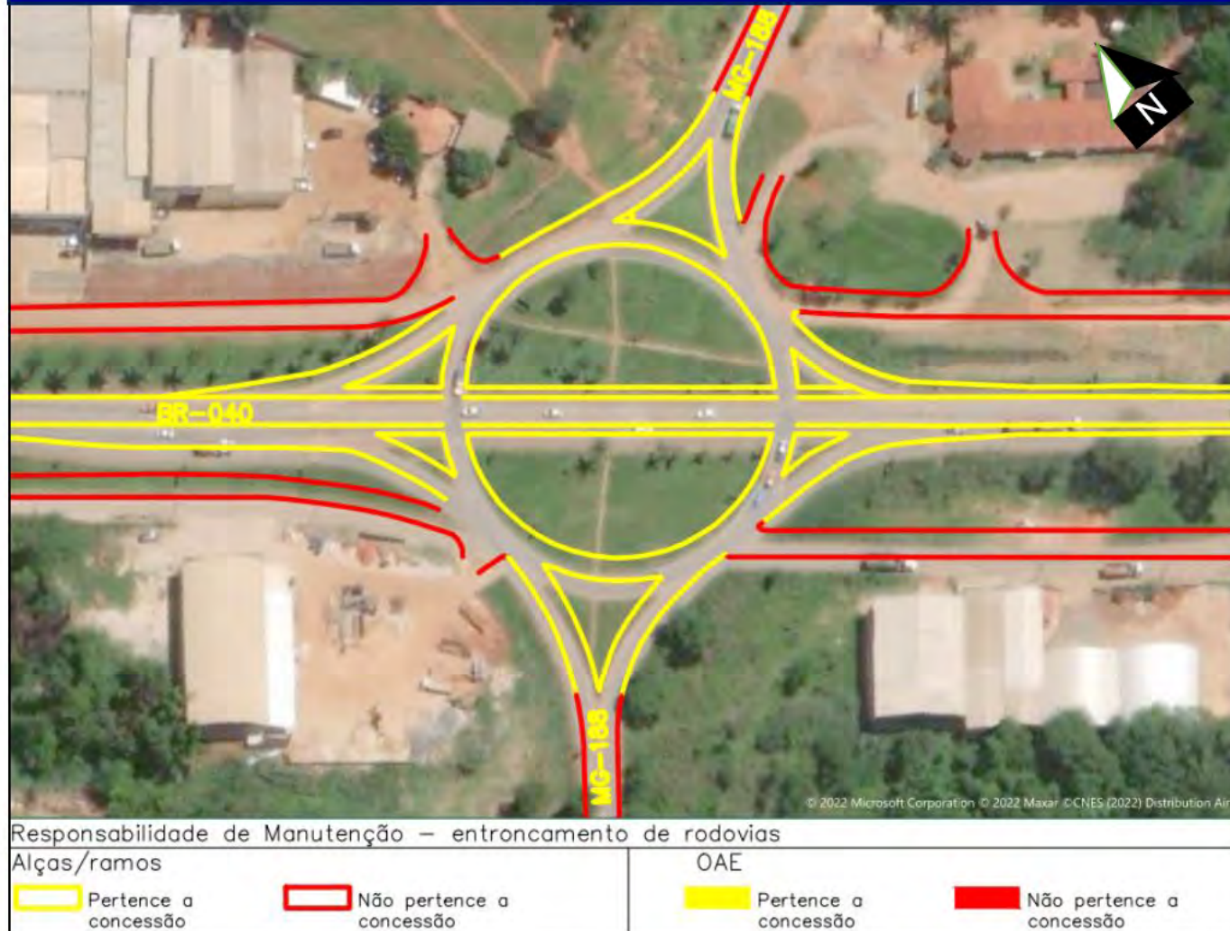
Figura 22 – Interseções BR-040/MG – Entroncamento com MG-188
