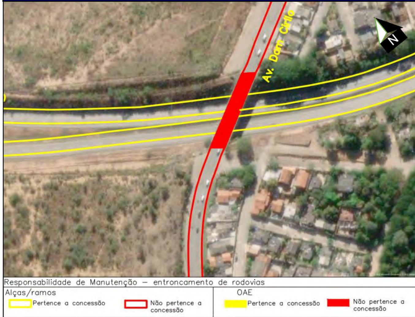
Figura 37 – Interseções BR-040/MG – Viaduto sobre BR-040
