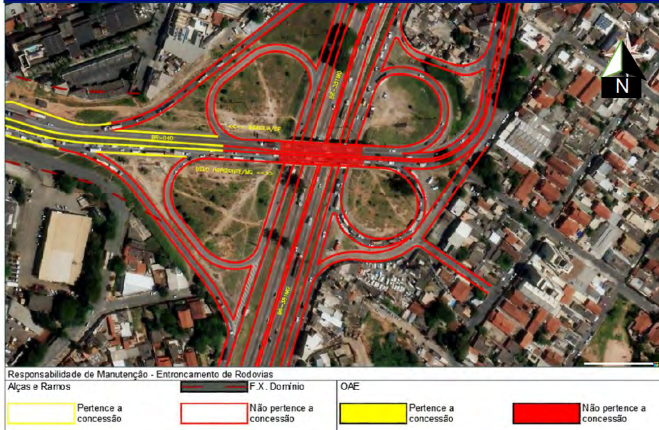
Figura 50 – Interseções BR-040/MG – Entroncamento com BR-381
