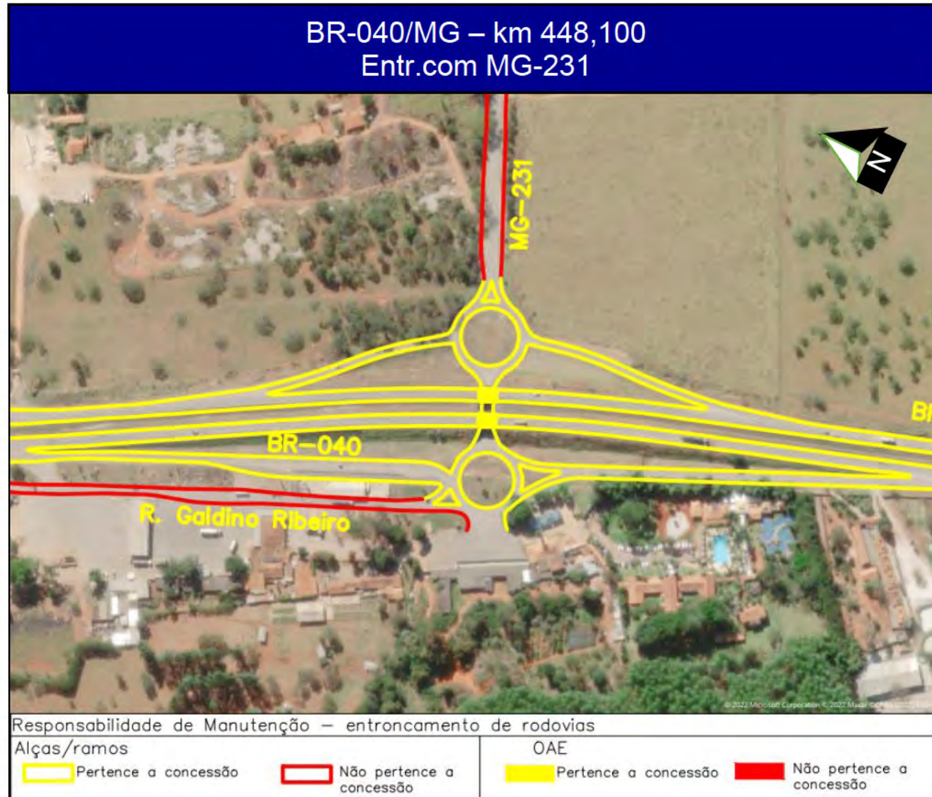
Figura 39 – Interseções BR-040/MG – Entroncamento com MG-231
