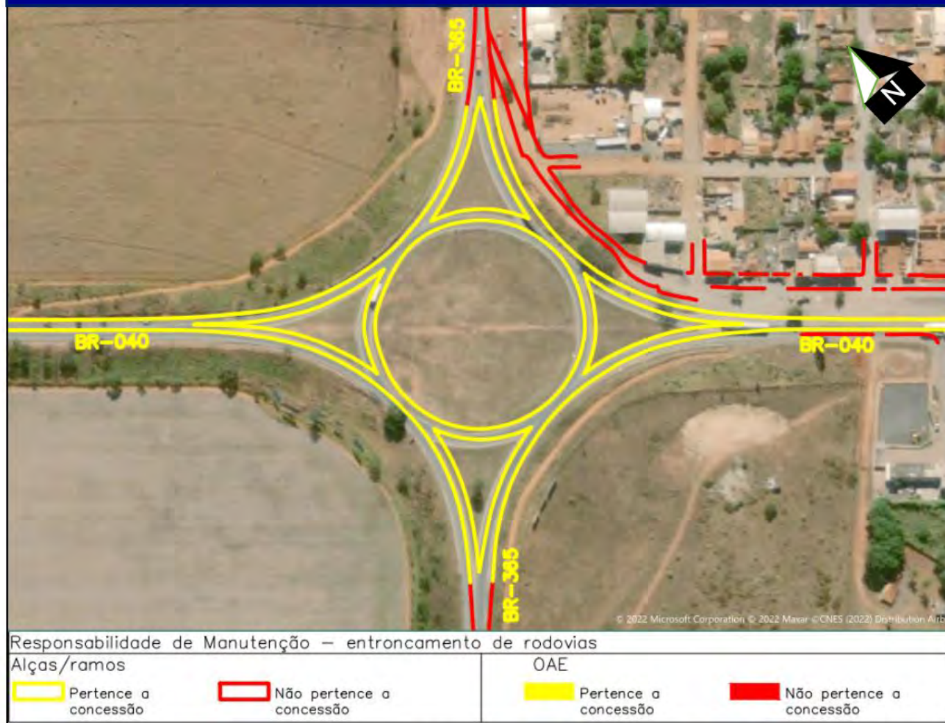
Figura 27 – Interseções BR-040/MG – Entroncamento com BR-365
