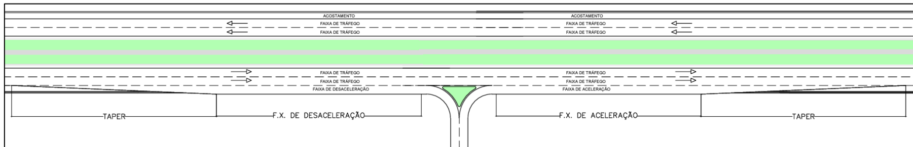
Figura 12 – Croqui Básico Acesso em Nível
