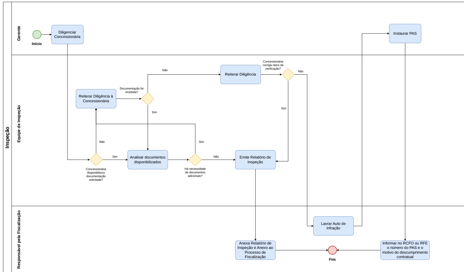
FIGURA D1 – Diagrama do Processo de “Realizar Inspeção”
