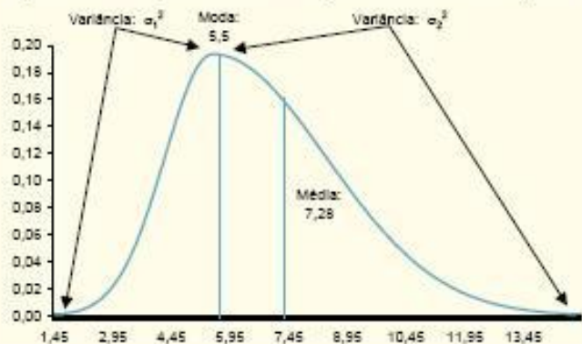
Figura 1 – Histograma da distribuição normal de duas partes
