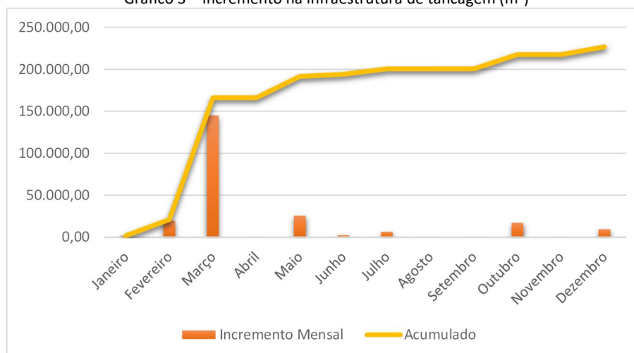
Gráfico 3 – Incremento na infraestrutura de tancagem (m 3 )
