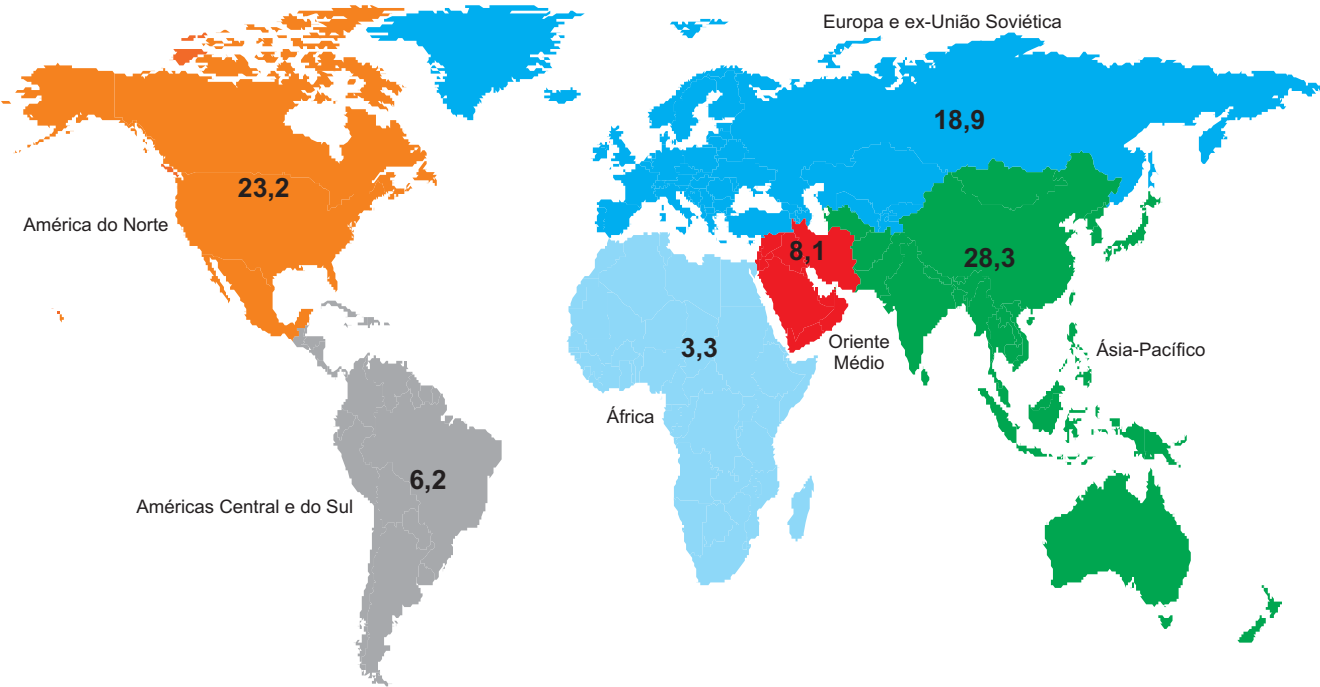
Cartograma 1.3 - Consumo de petróleo, segundo regiões geográficas em 2011 (milhões de barris/dia)
