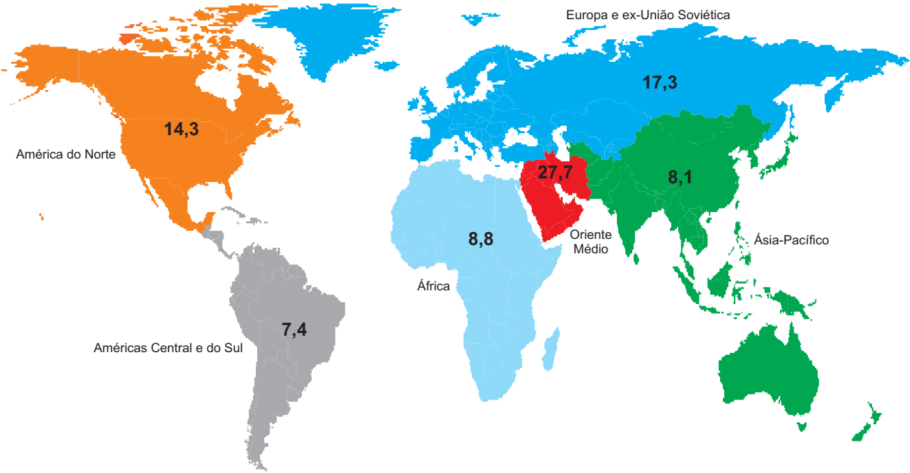
Cartograma 1.2 - Produção de petróleo, segundo regiões geográficas em 2011 (milhões de barris/dia)
