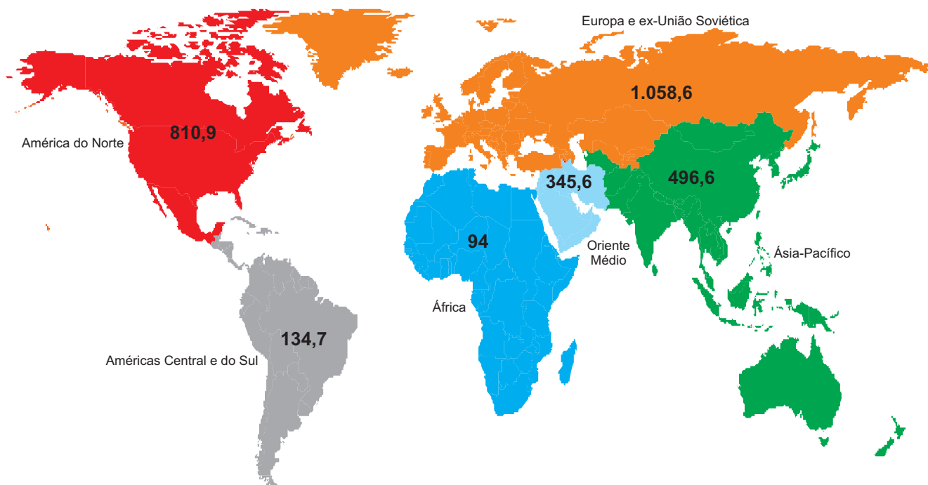
Cartograma 1.7 - Consumo de gás natural, segundo regiões geográficas em 2009 (bilhões m 3 )
