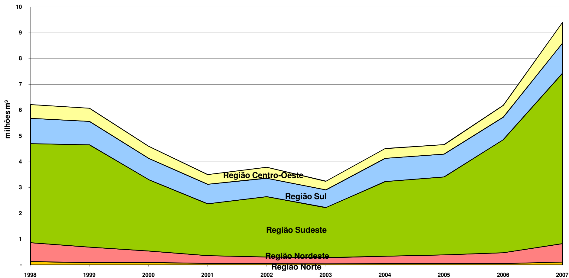
Gráfico 4.7 - Evolução das vendas, pelas distribuidoras, de álcool etílico hidratado, segundo Grandes Regiões - 1998-2007
