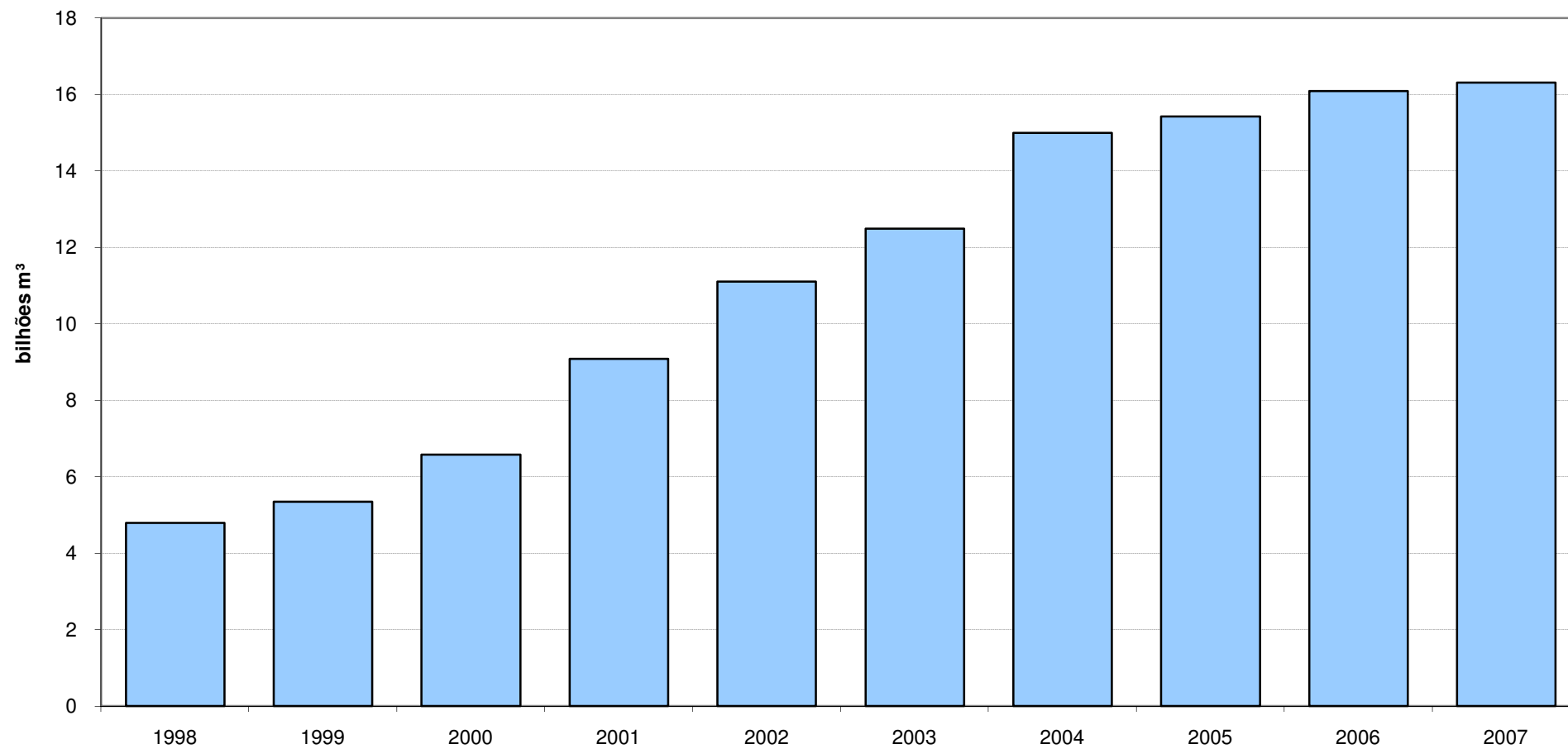
Gráfico 3.13 - Evolução das vendas nacionais, pelos produtores, de gás natural - 1998-2007
