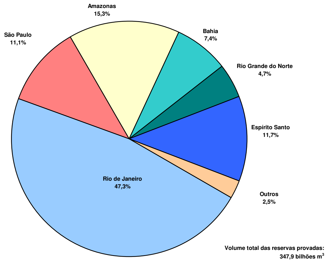
Gráfico 2.4 - Distribuição percentual das reservas provadas de gás natural, segundo Unidades da Federação, em 31/12/2006
