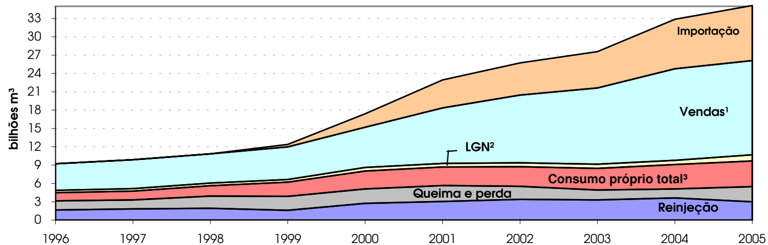
Gráfico 3.12 - Evolução do balanço do gás natural no Brasil - 1996-2005
