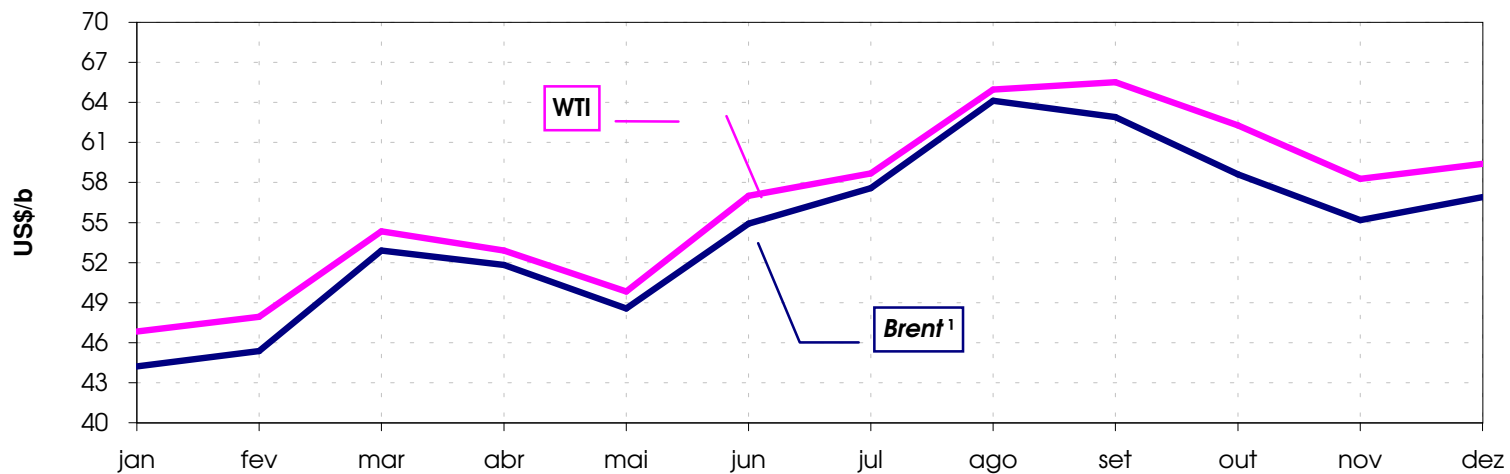
Gráfico 1.5 - Evolução dos preços médios mensais no mercado spot dos petróleos dos tipos Brent e West Texas Intermediate (WTI) - 2005
