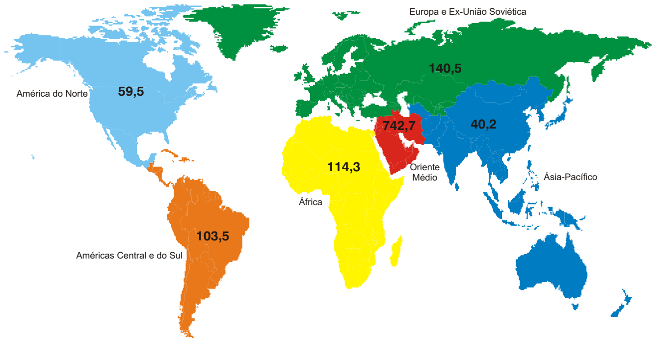
Cartograma 1.1 - Reservas provadas de petróleo, segundo regiões geográficas, em 31/12/2005 (bilhões b)
