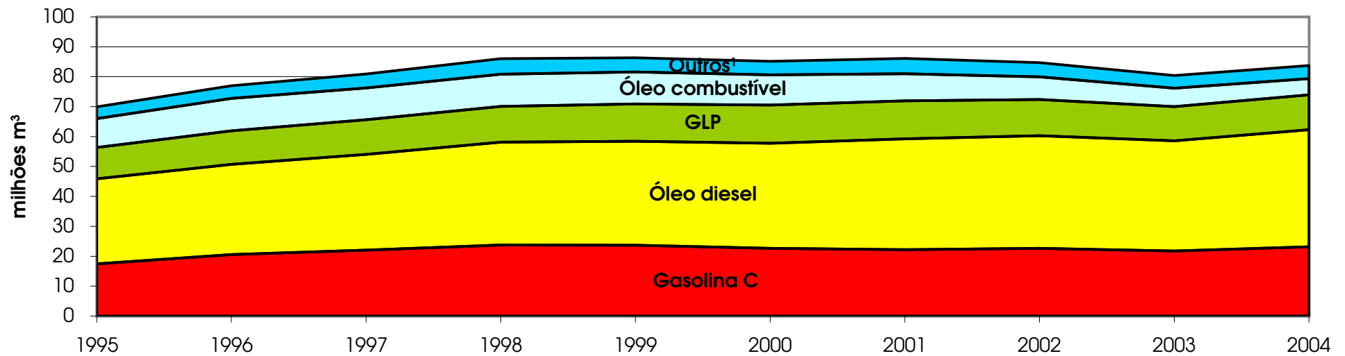
Gráfico 3.1 - Evolução das vendas nacionais, pelas distribuidoras, dos principais derivados de petróleo - 1995-2004
