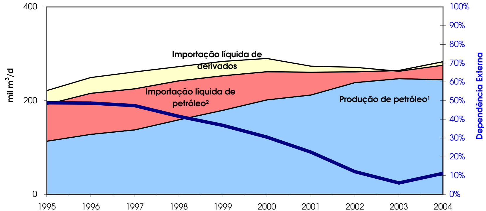
Gráfico 2.24 - Evolução da dependência externa de petróleo e seus derivados - 1995-2004
