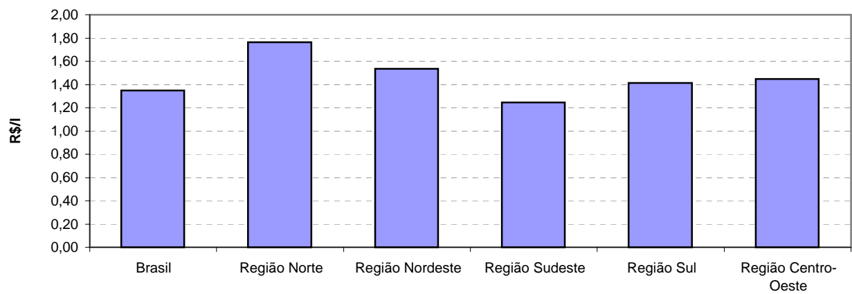
Gráfico 4.9 - Preço médio de álcool etílico hidratado ao consumidor, segundo Grandes Regiões - 2003
