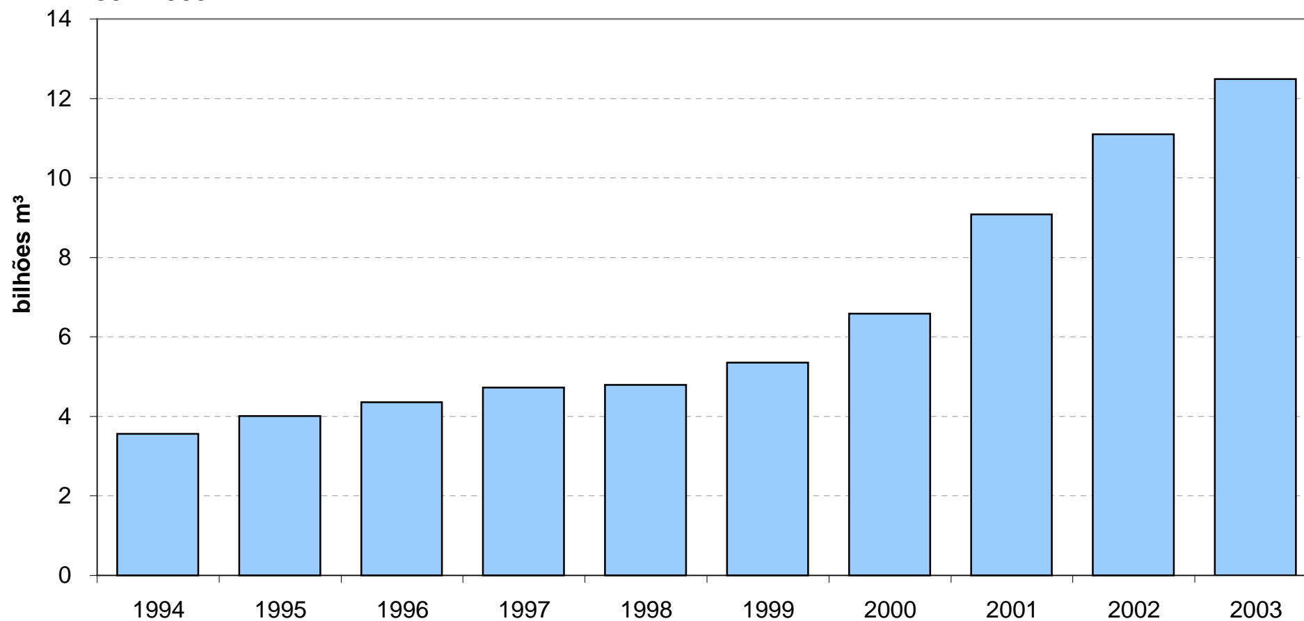
Gráfico 3.13 - Evolução das vendas nacionais, pelos produtores, de gás natural - 1994-2003
