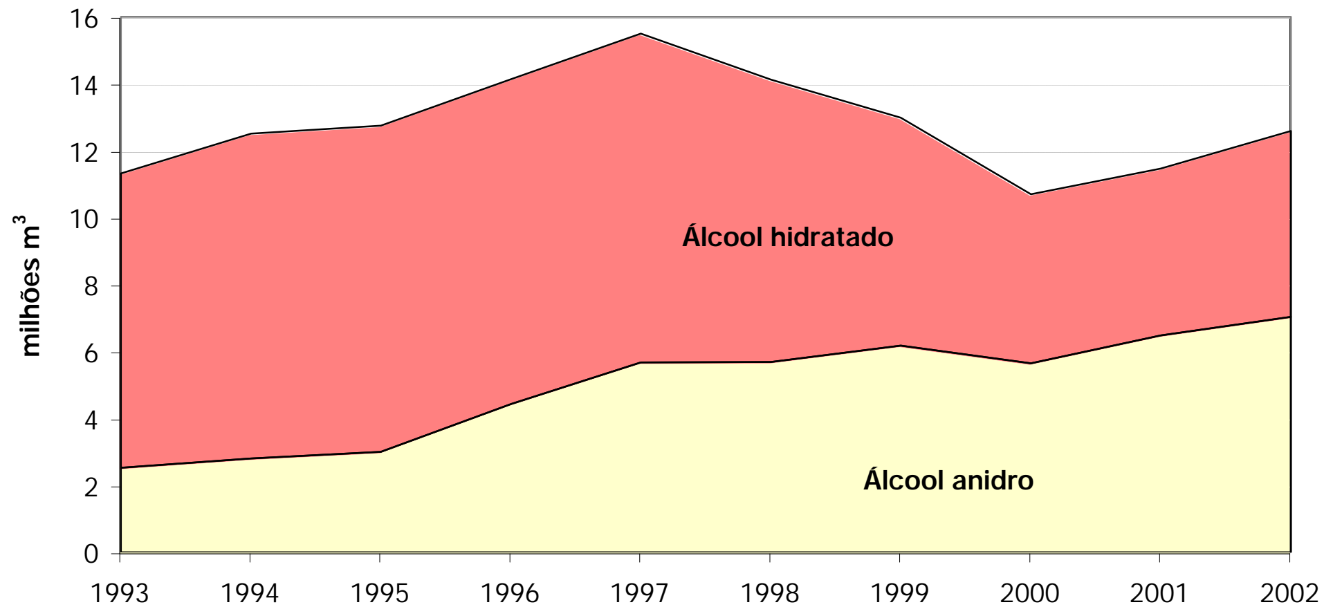
Gráfico 4.2 - Evolução da produção nacional de álcool etílico anidro e hidratado - 1993-2002
