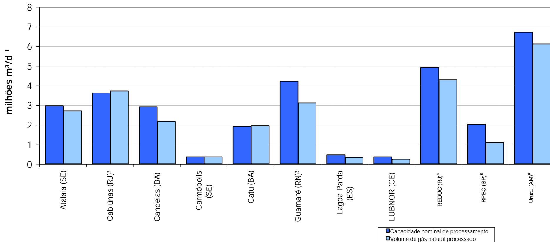
Gráfico 2.13 - Volume de gás natural processado e capacidade nominal de processamento, segundo UPGNs - 2002
