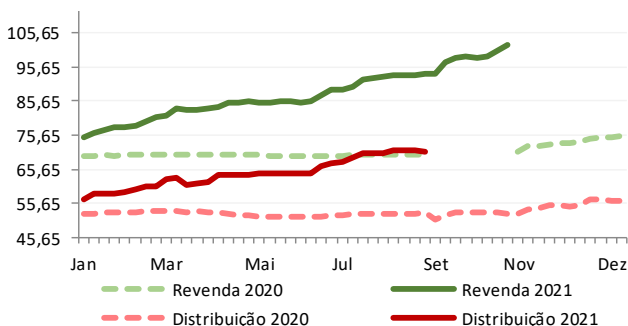
Preços semanais de revenda e distribuição de GLP P-13 (média nacional) - 2020/2021
