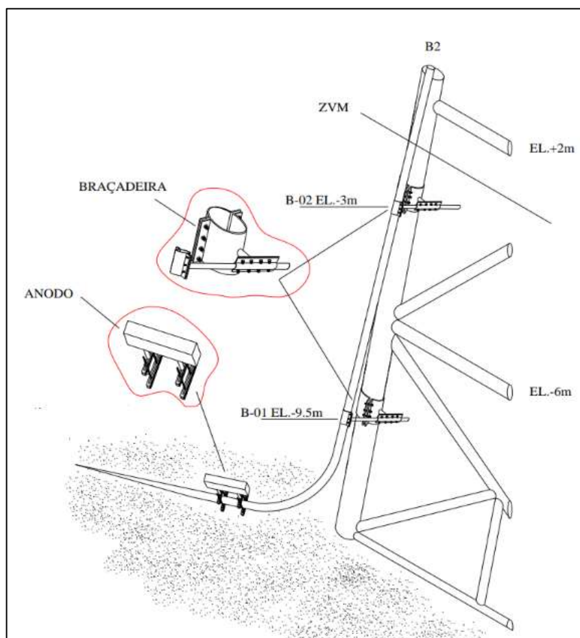
Figura 3-II: Desenho esquemático para ilustrar a forma de fixação de cada riser na jaqueta PAG-01
