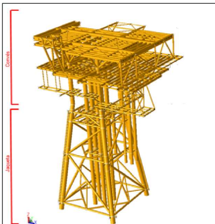
Figura 3.2.3-I: Arranjo geral da jaqueta da PAG-01
