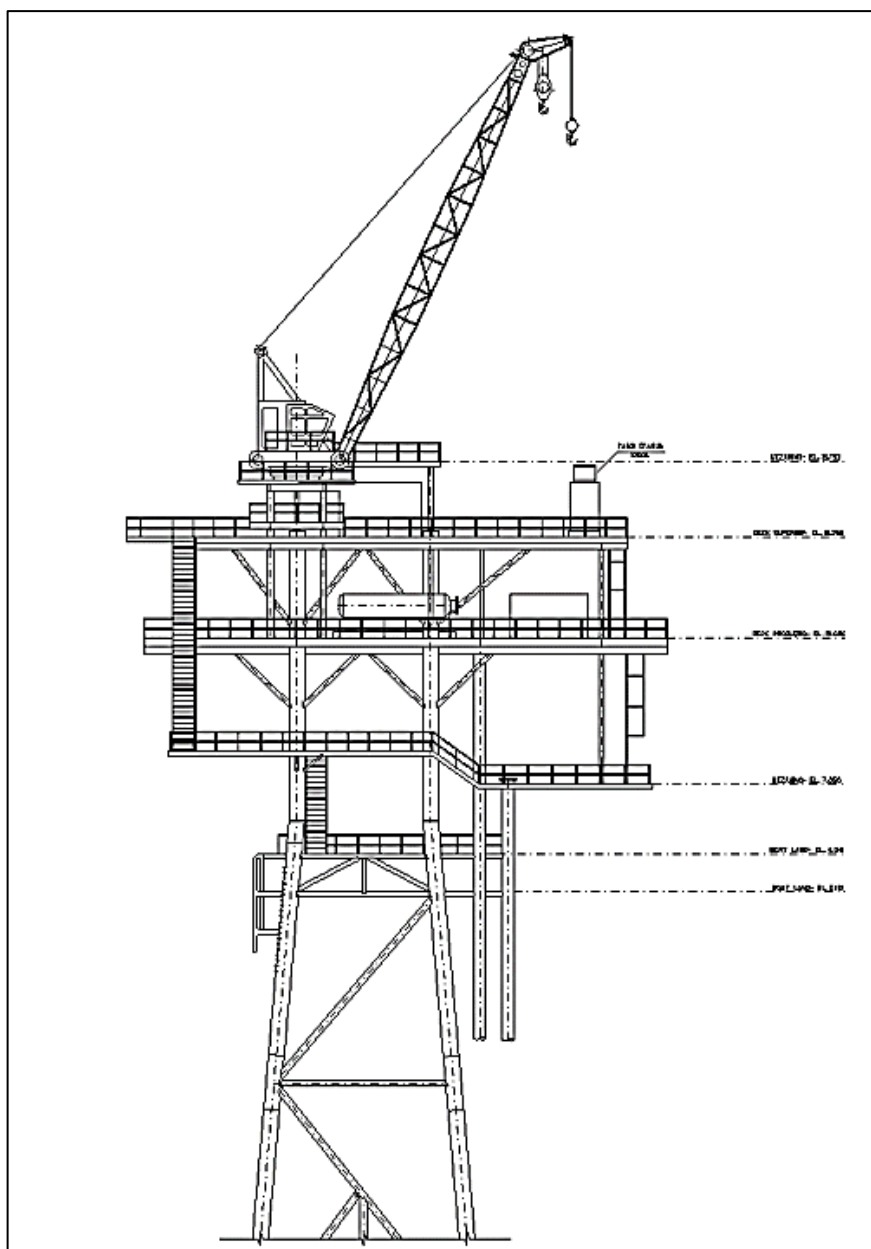
Figura 3.2.2-I: Arranjo geral da jaqueta e conveses da PAG-01.
