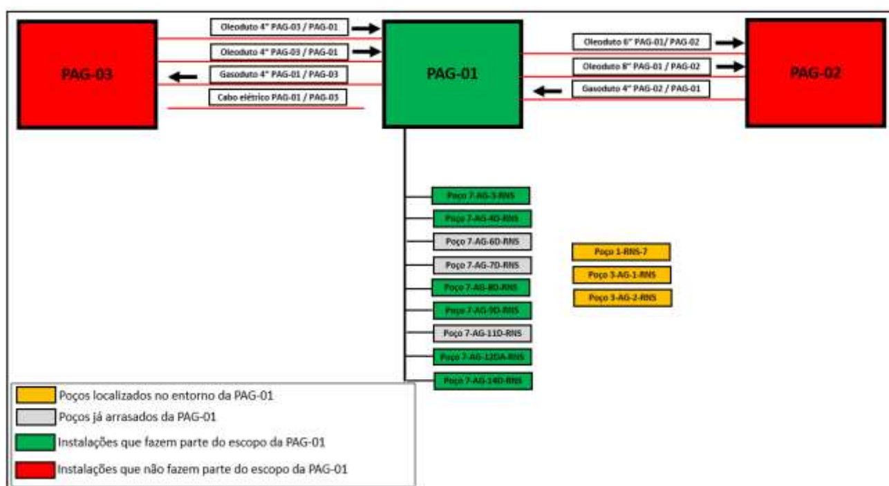
Figura 3-I: Sistema de dutos submarinos associados ao escopo completo da PAG-01.
