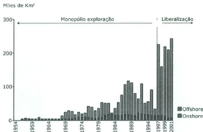
Figura III.40: Evolução da área explorada através de exploração sísmica no Brasil
