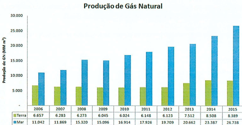
Figura 6. Produção de gás natural, por localização (terra e mar) - 2006-2015. Fonte: ANP.
