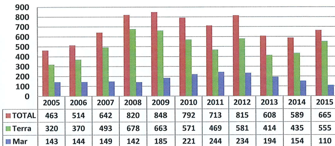
Figura 3. Poços perfurados, por localização (terra e mar). Fonte: ANP.
