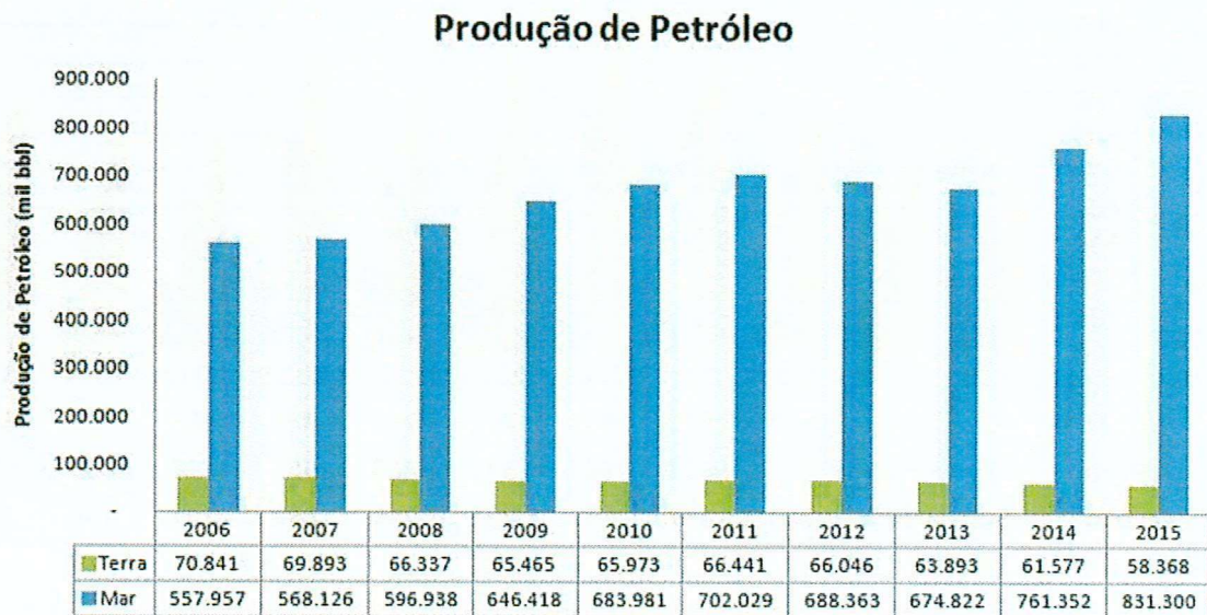
Figura 5. Produção de petróleo, por localização (terra e mar) - 2006-2015. Fonte: ANP.
