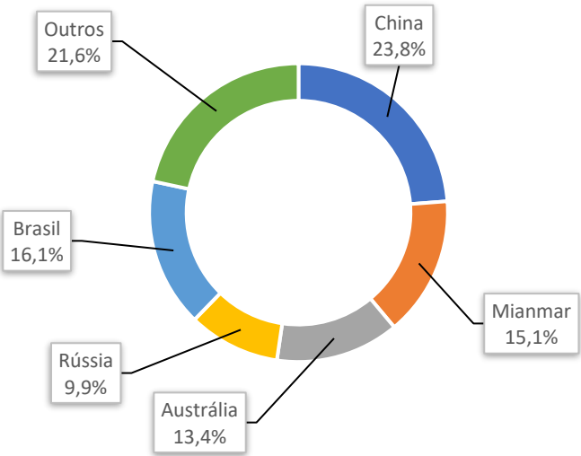
Fonte: Mundo: USGS Mineral Commodity Summaries 2024. Brasil: ANM FIGURA 1 – Principais Reservas Mundiais de Estanho – 2023
