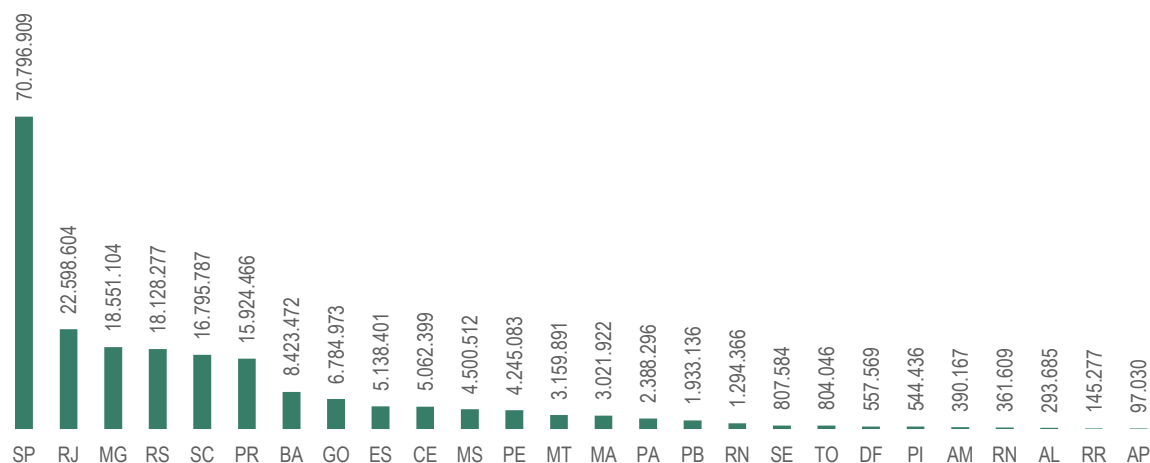
Figura 02- Quantidade produzida, em toneladas, de rocha britada por Unidade da Federação.
