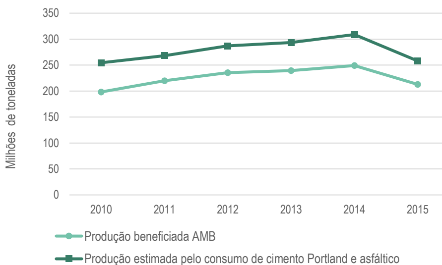
Figura 04 – Comparação entre os dados de produção nacional de brita declarados no RAL/AMB e aqueles estimados a partir do consumo de cimento e asfalto para o período 2010 – 2015.
